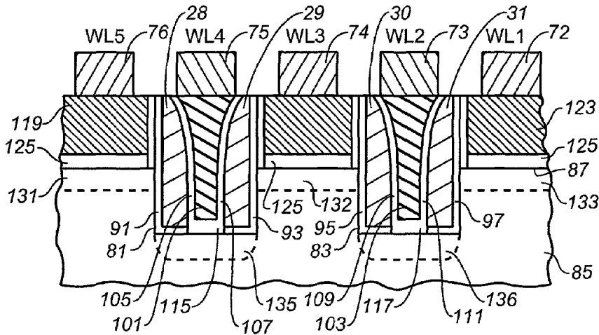
FIG. 3 (Section A-A)
