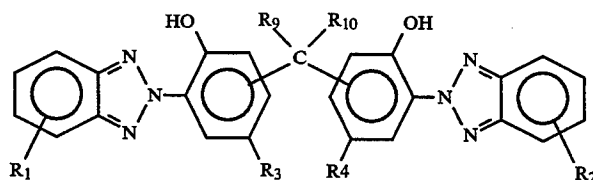
Compound 1-a
