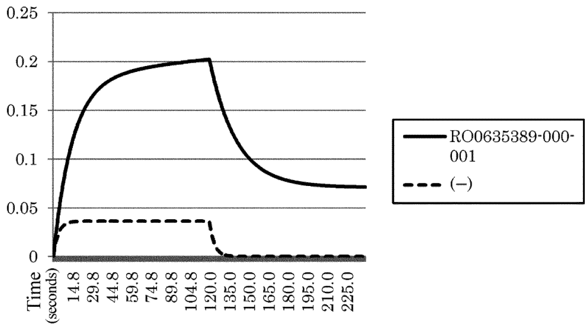
FIG. 28
