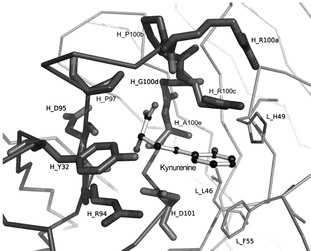
FIG. 34
