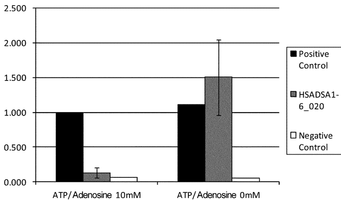
FIG. 46
