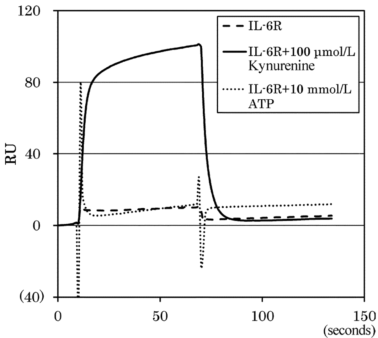
FIG. 19
