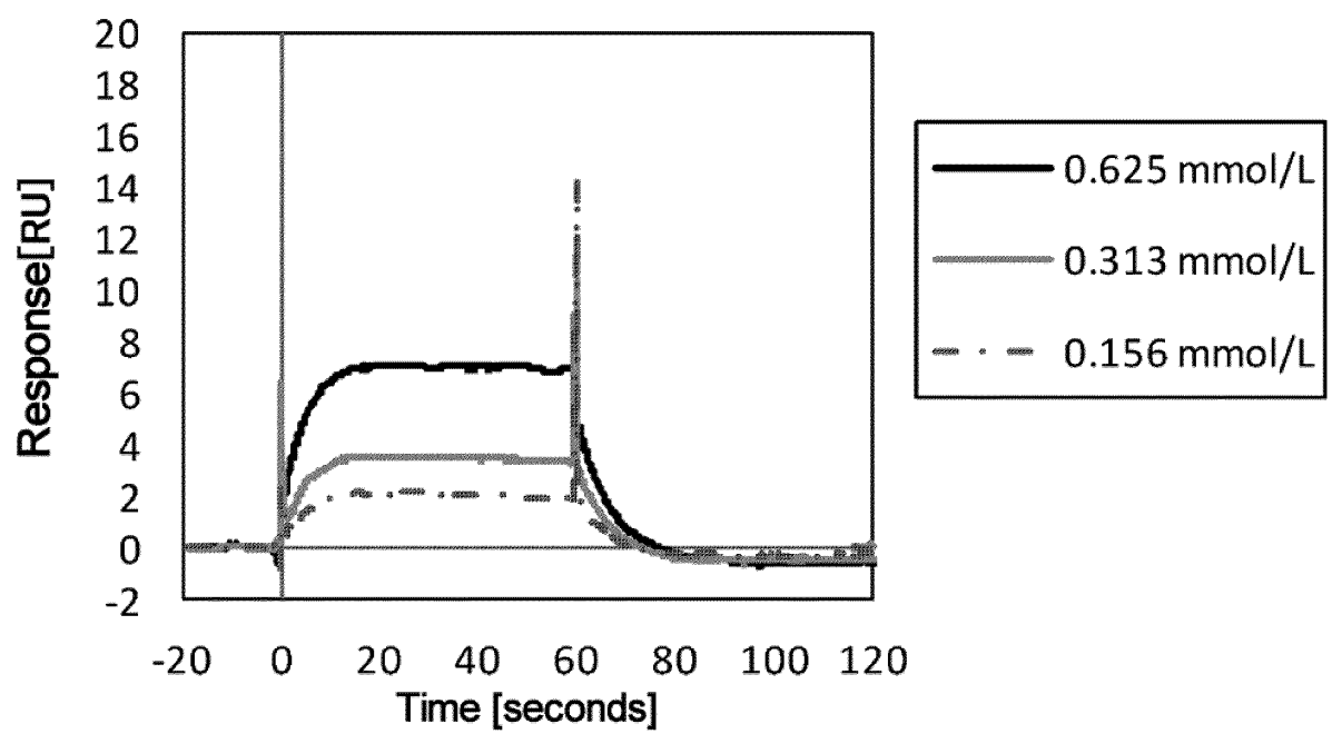
FIG. 25
