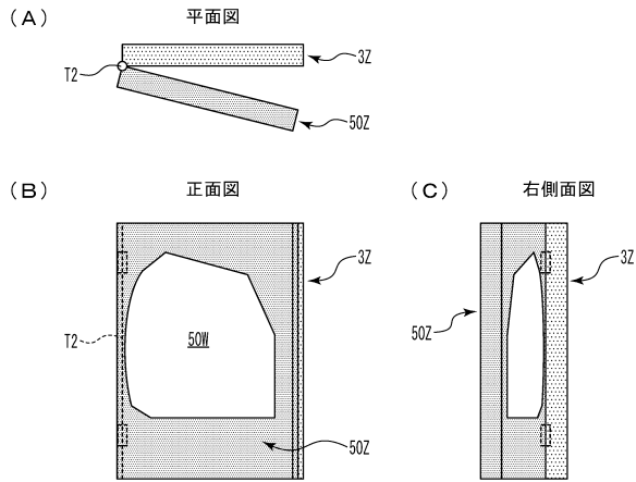
【図13-38】 開閉扉枠の開放態様 [垂れ下がりがなし]
