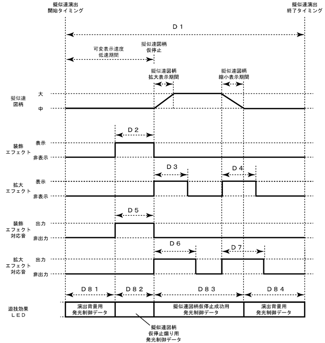
【図9-112】 擬似連演出
