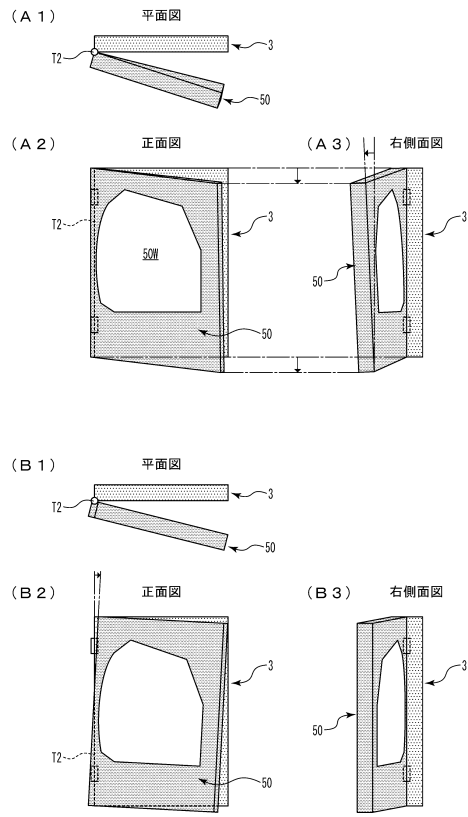
【図13-39】 開閉扉枠の開放態様 [垂れ下がりがあり]
