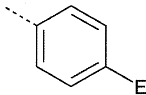
Formule (III)
