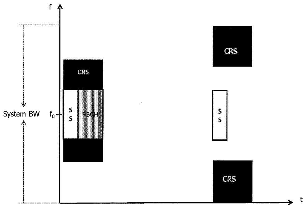
FIG. 3g
