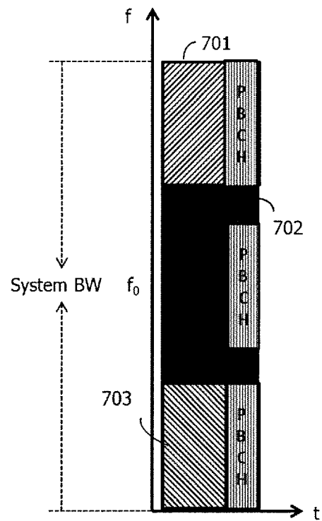
FIG. 7b
