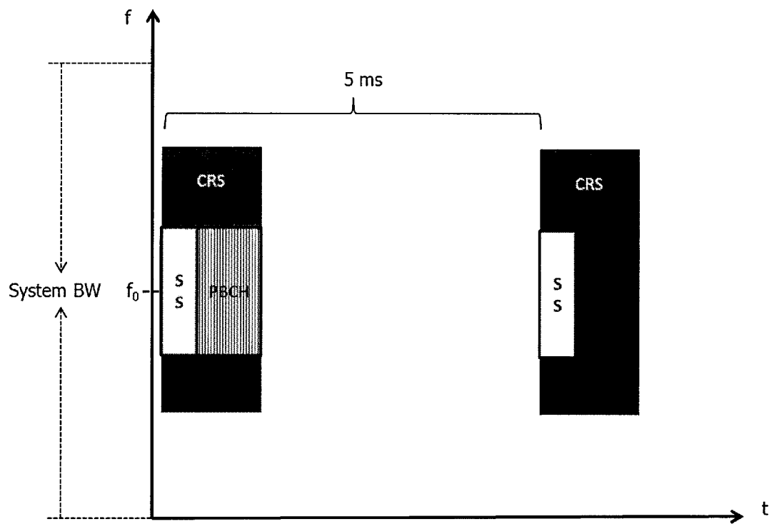
FIG. 3e
