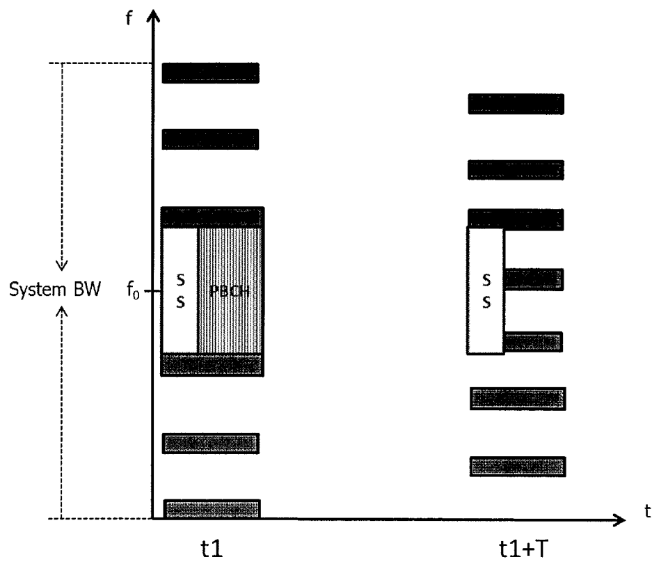
FIG. 3f
