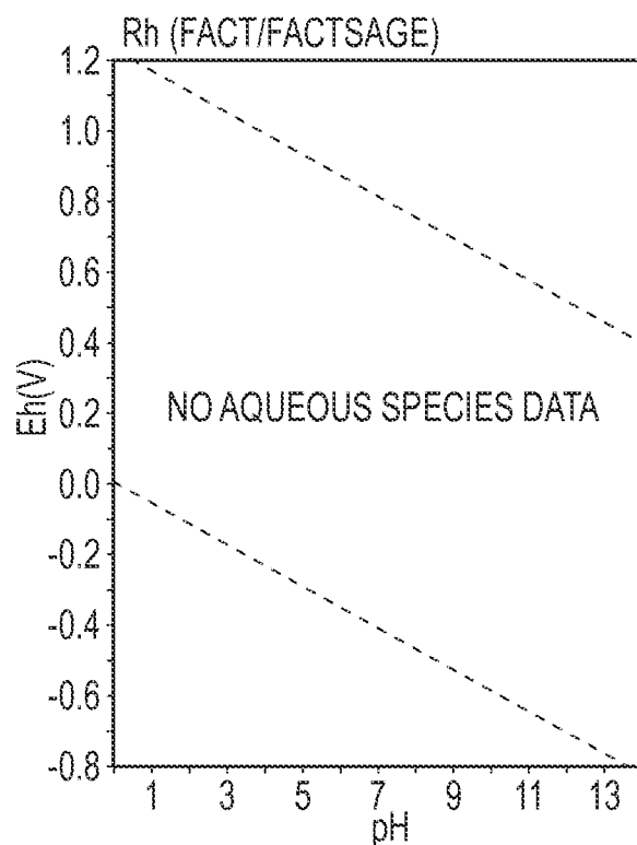
FIG. 21A PRIOR ART
