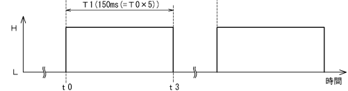
(e) TD点の論理
