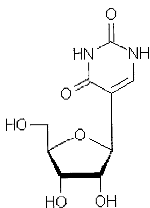
Pseudouridine(Ψ)
