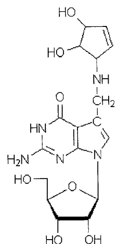
Queuosine(Q)
