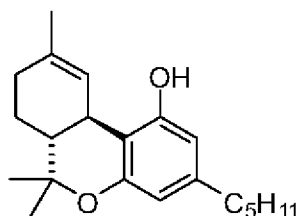
THC
