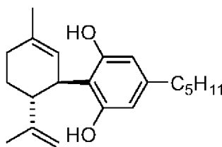
CBD
