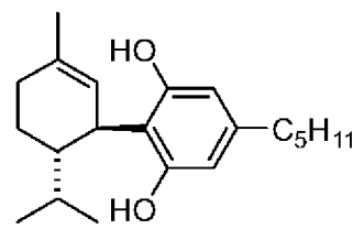
H2CBD
