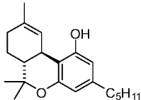
THC
