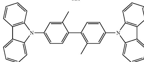
CDBP
