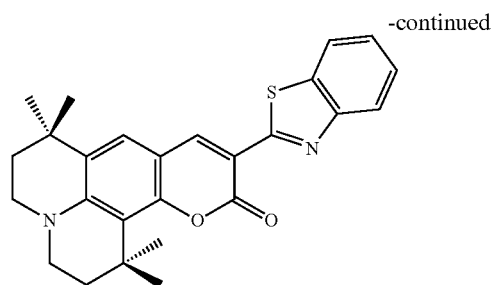
C545T
