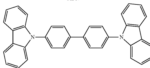
CBP
