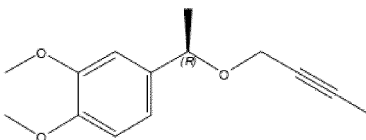
( R )-4-(1-(but-2-ynoxy)ethyl)-1,2-dimethoxybenzene (Formula XV)
