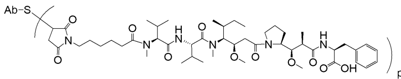
Ab-MC-MMAF
