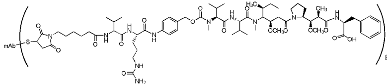
L-MC-vc-PAB-MMAE.
