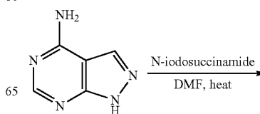
Scheme I.
