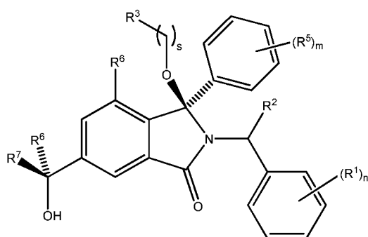
Diastereoisomer 2A
