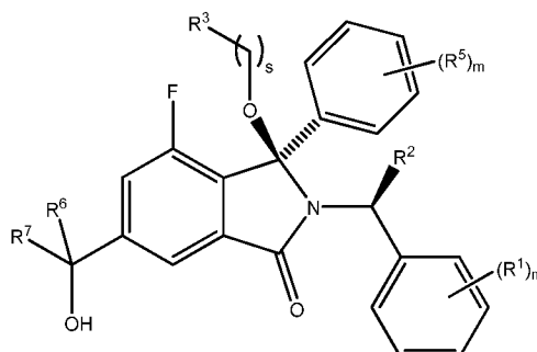
Diastereoisomer 1A
