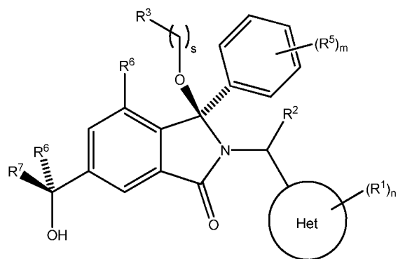
Diastereoisomer 2A
