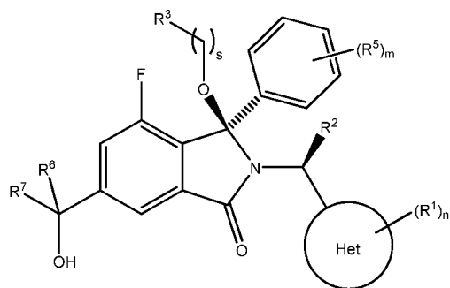
Diastereoisomer 1A
