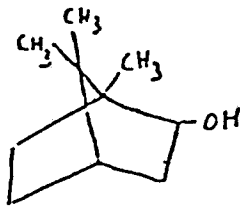
Borneol
