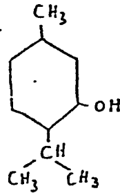
Menthol
