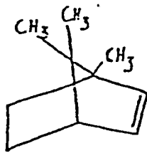
Bornen
