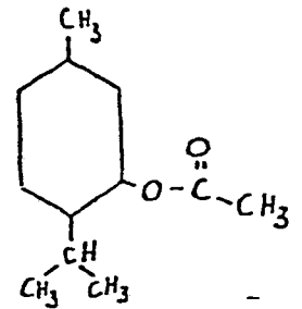
Menthylacetat
