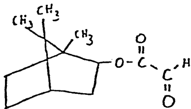
Bornylglyoxylat
