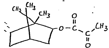
Bornylpyruvat
