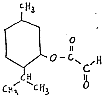
Menthylglyoxylat
