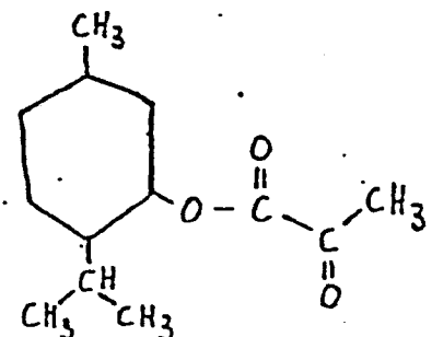
Menthylpyruvat
