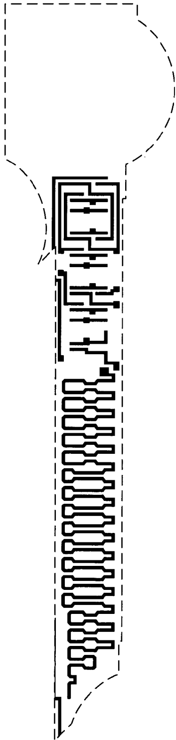
Poly mask
