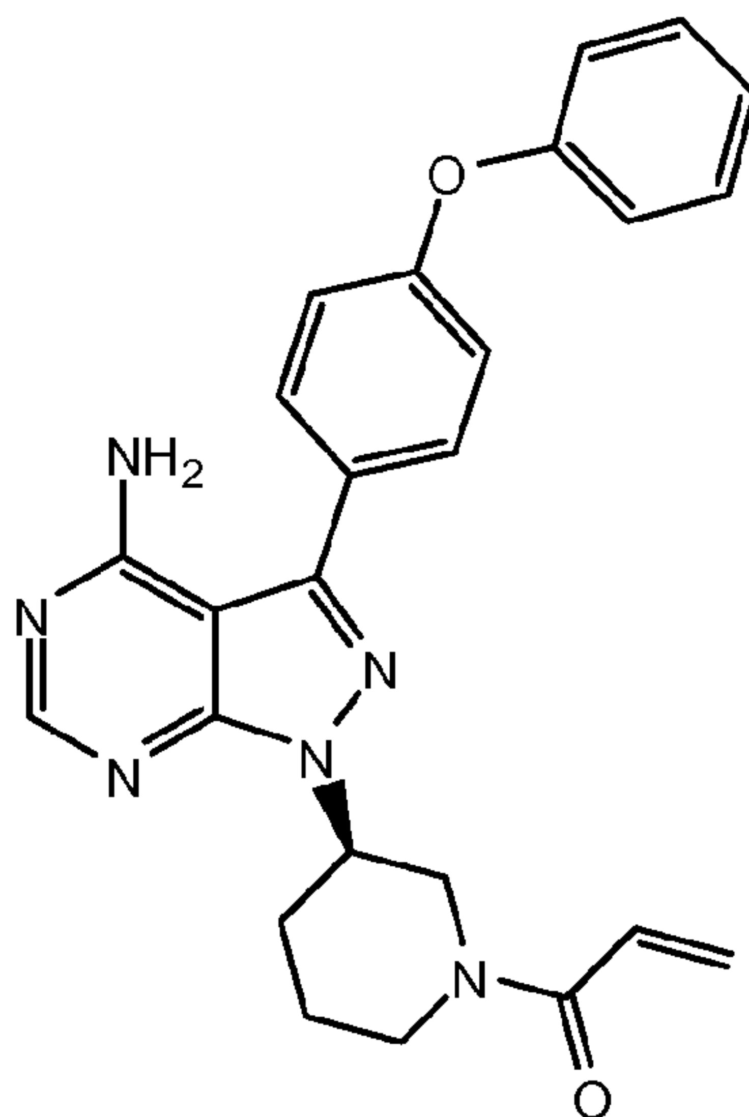
Ibrutinib.
