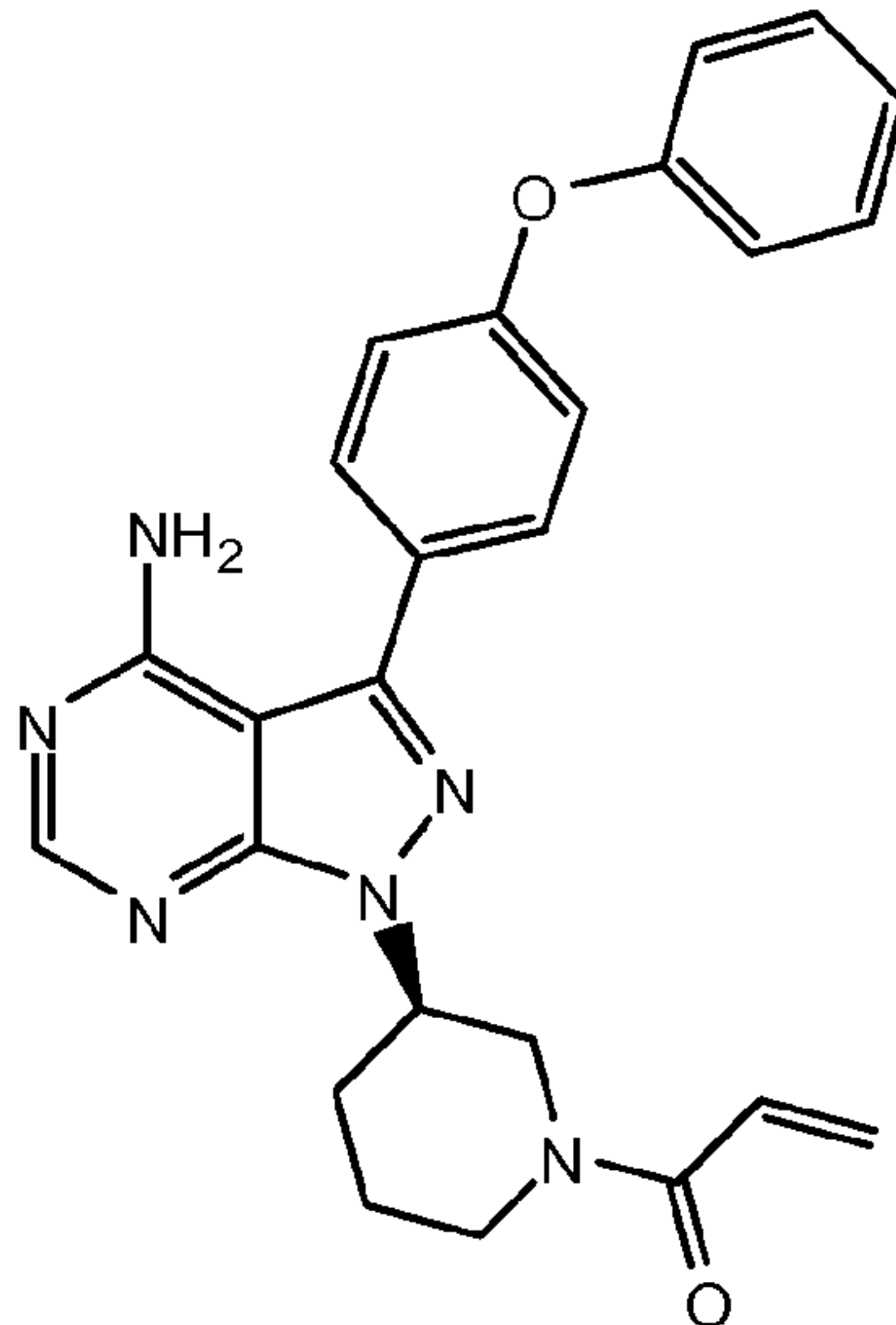
Ibrutinib.
