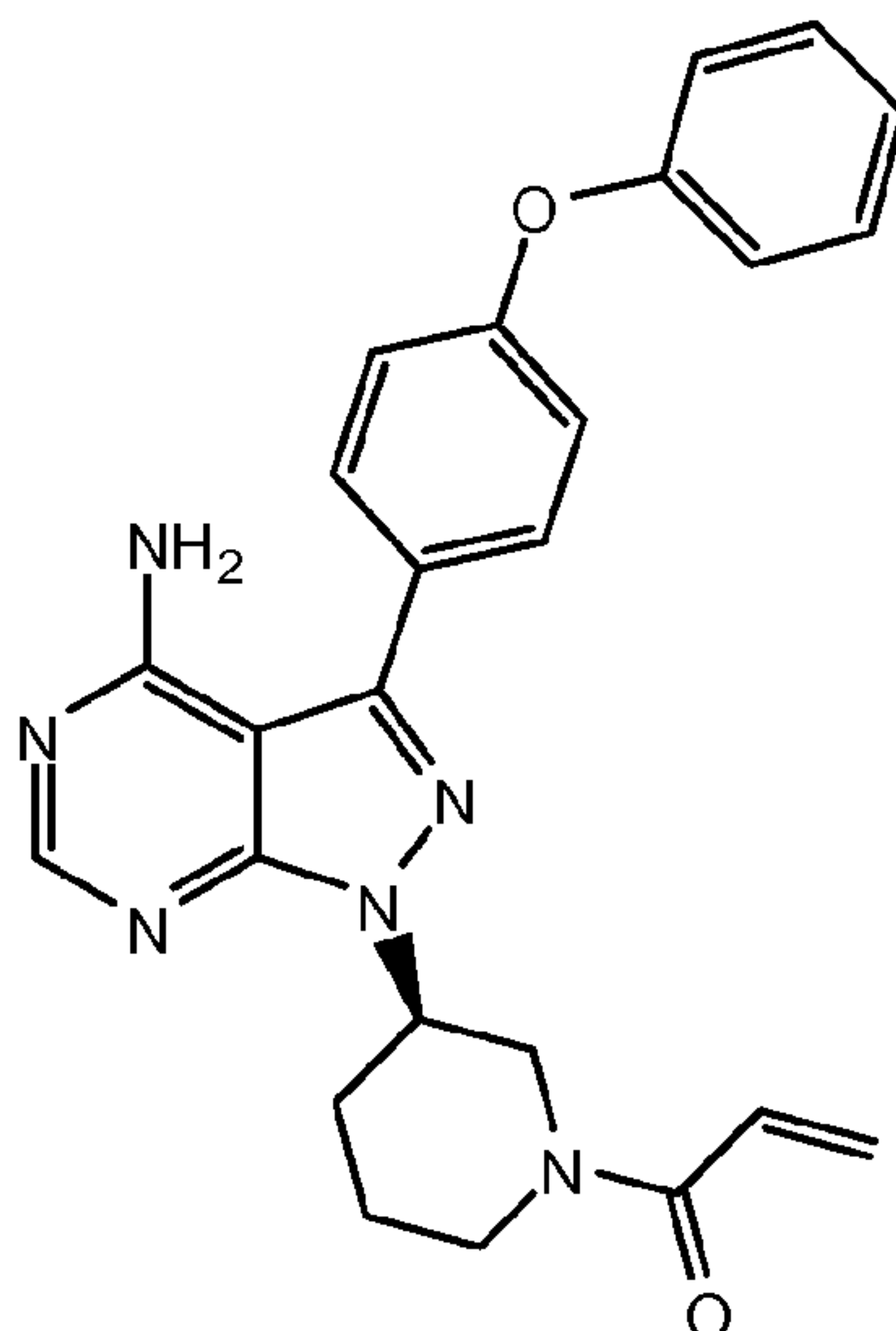
Ibrutinib.
