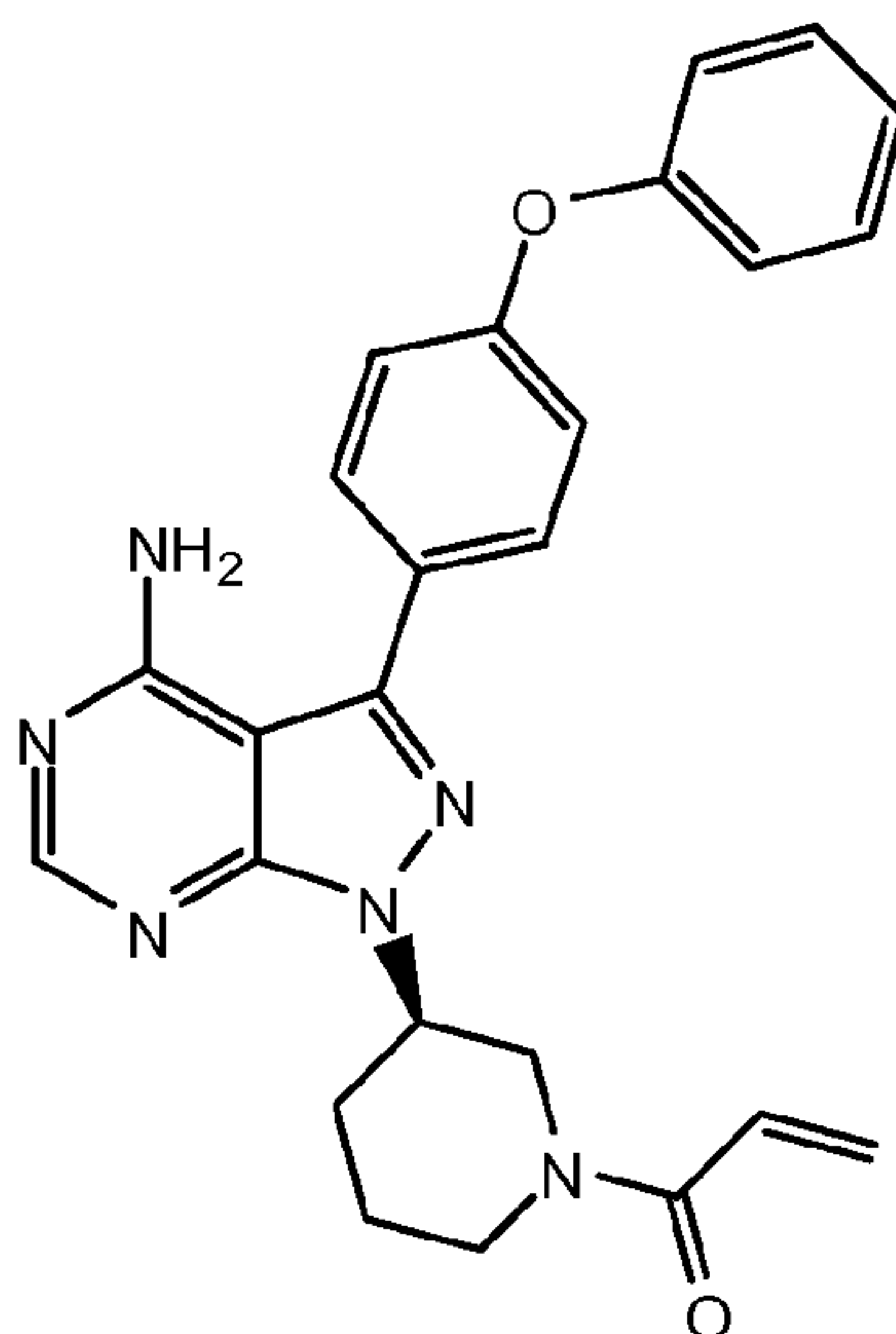
Ibrutinib.
