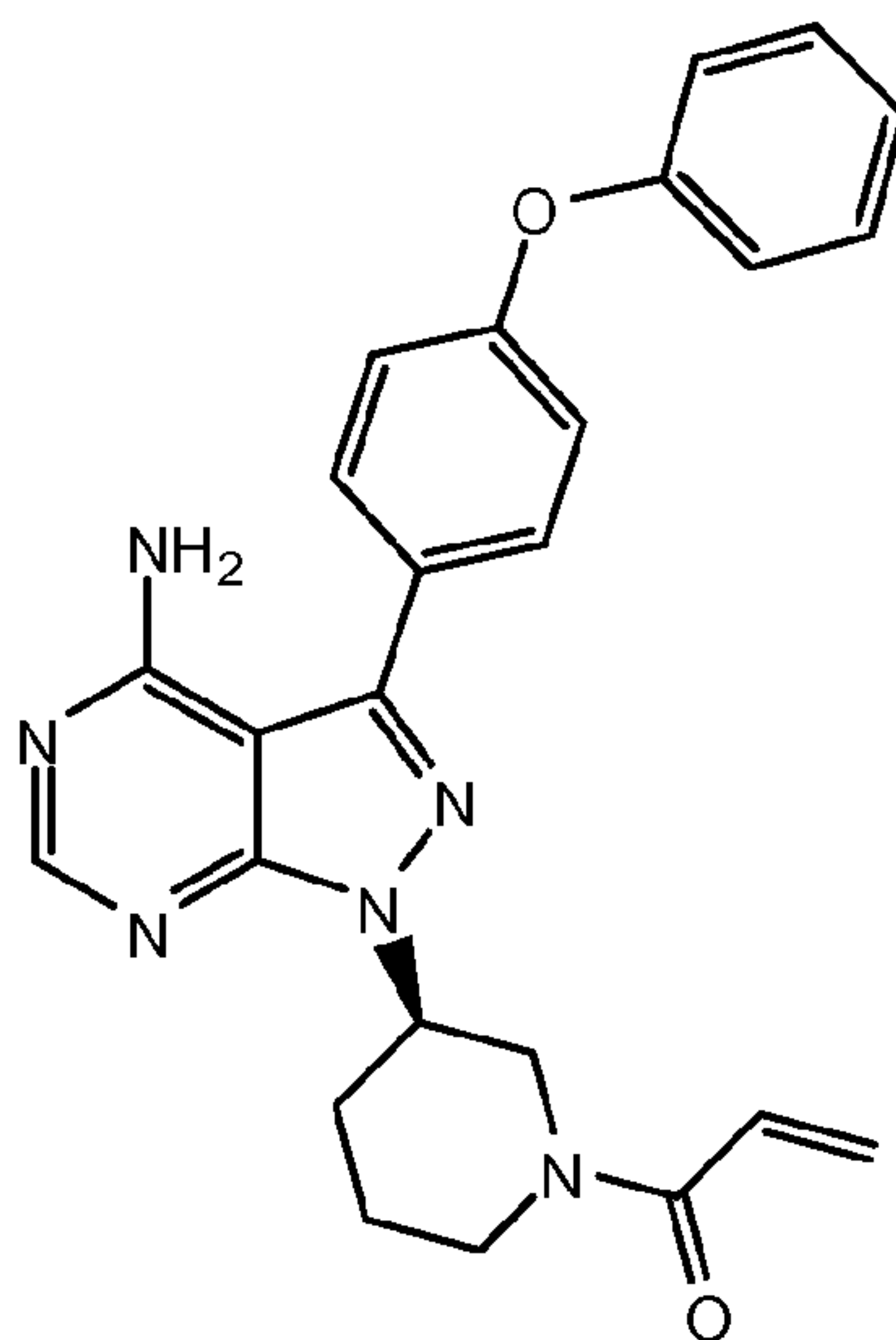
Ibrutinib.
