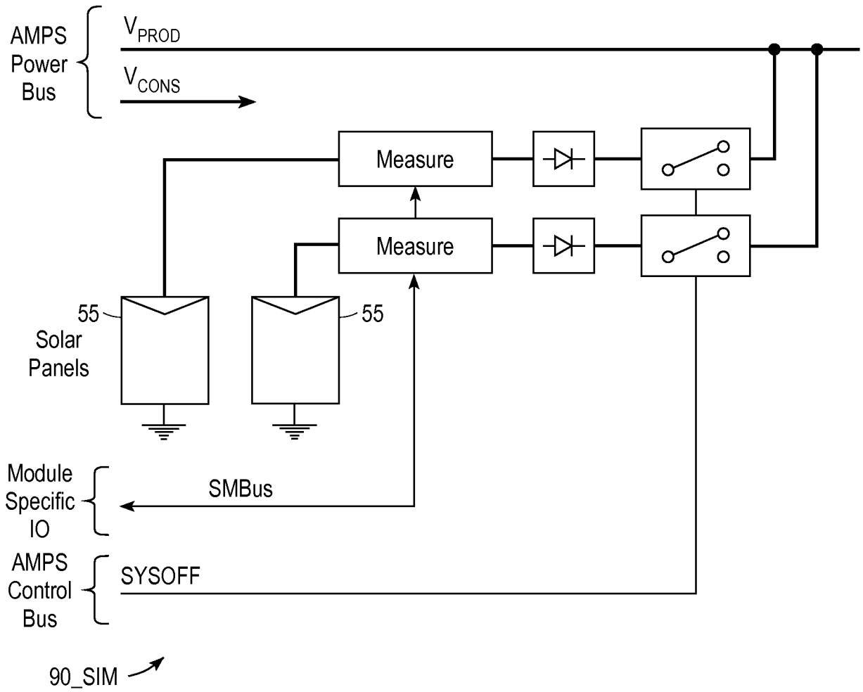
FIG. 13 – Solar Input Module
