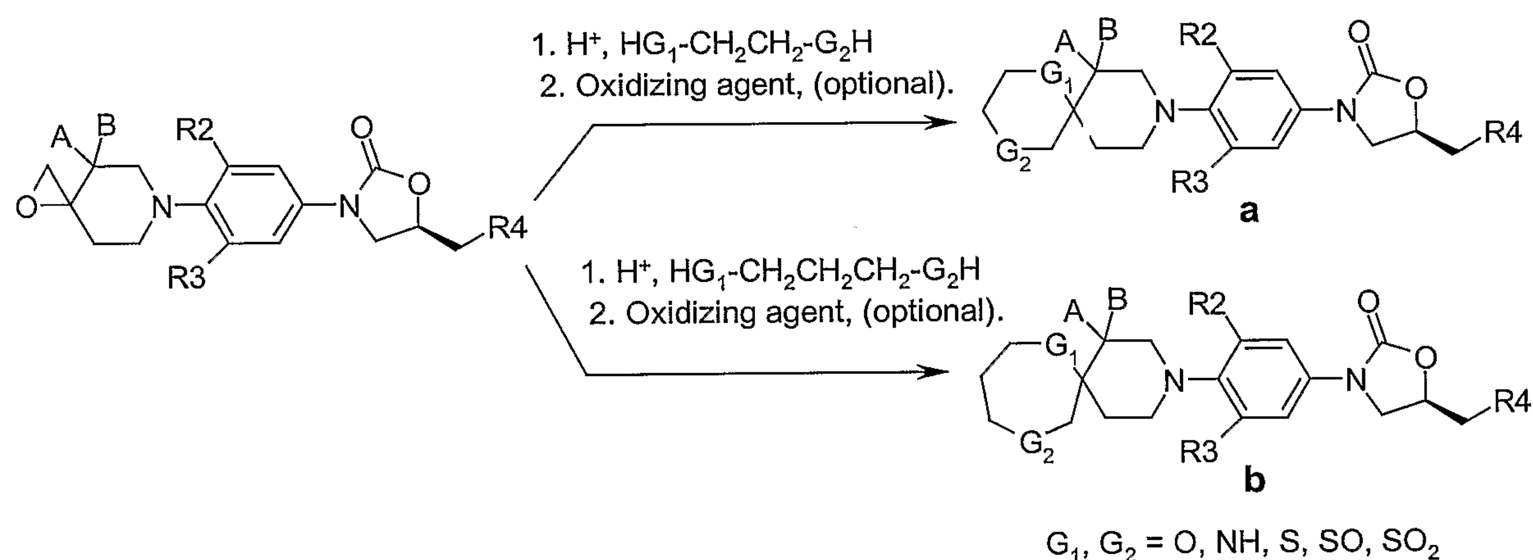
Scheme-5
