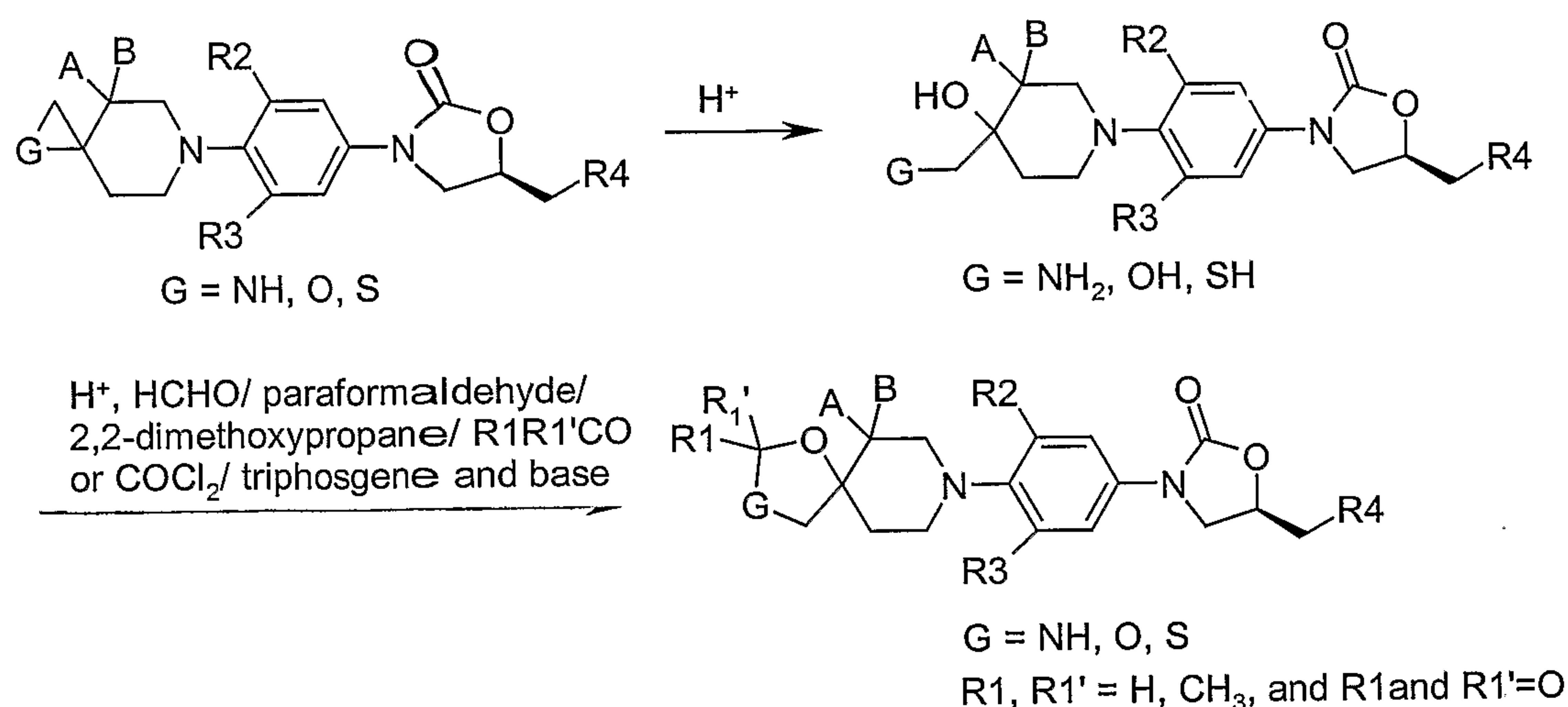
Scheme-4
