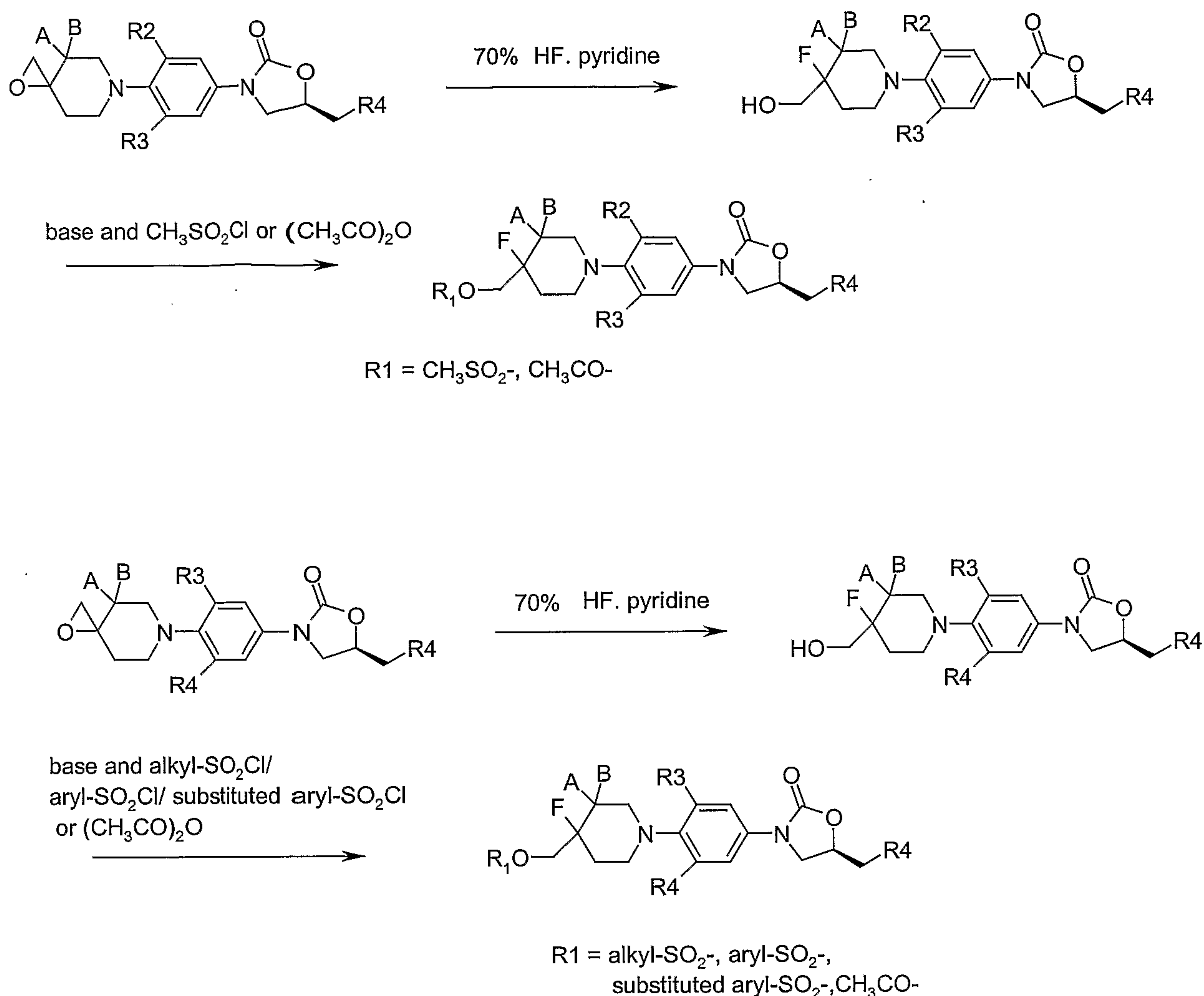
Scheme-12
