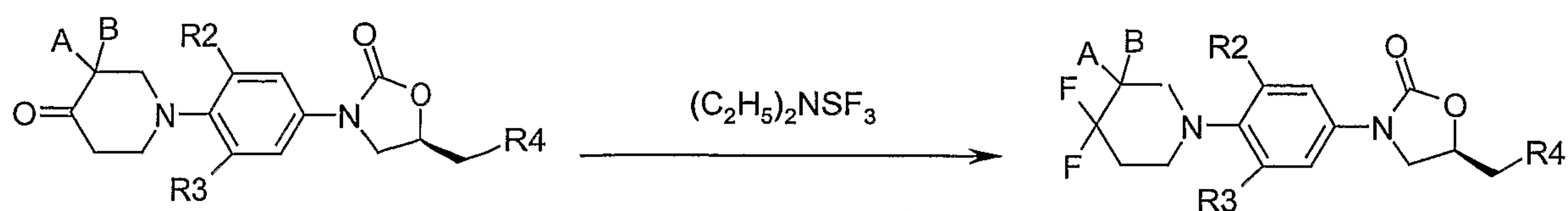
Scheme-10
