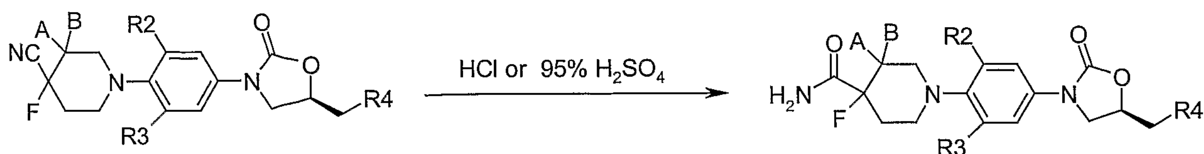
Scheme-13
