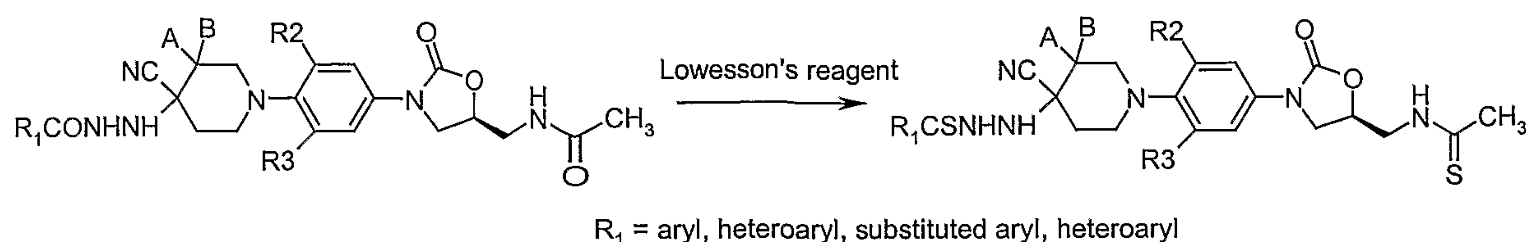
Scheme-20
