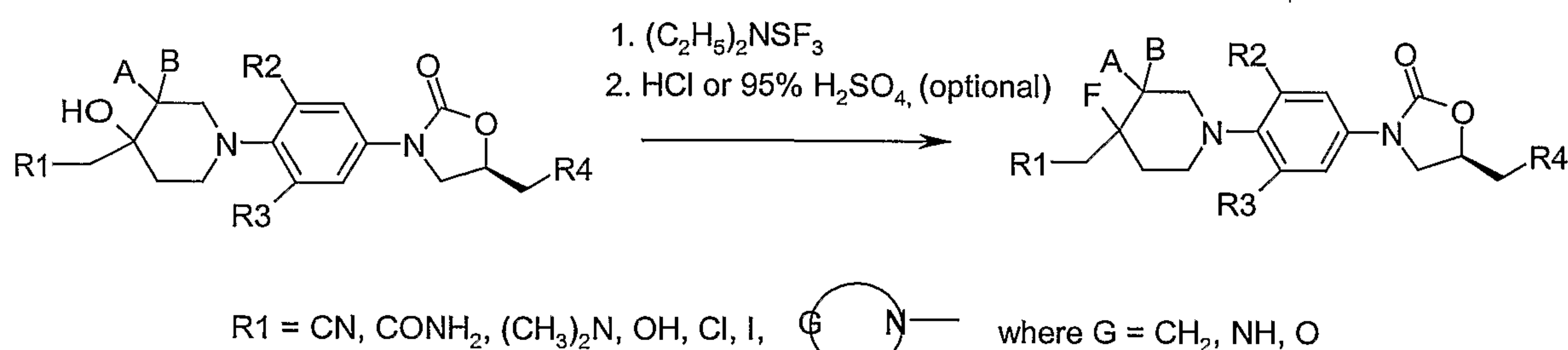
Scheme-11
