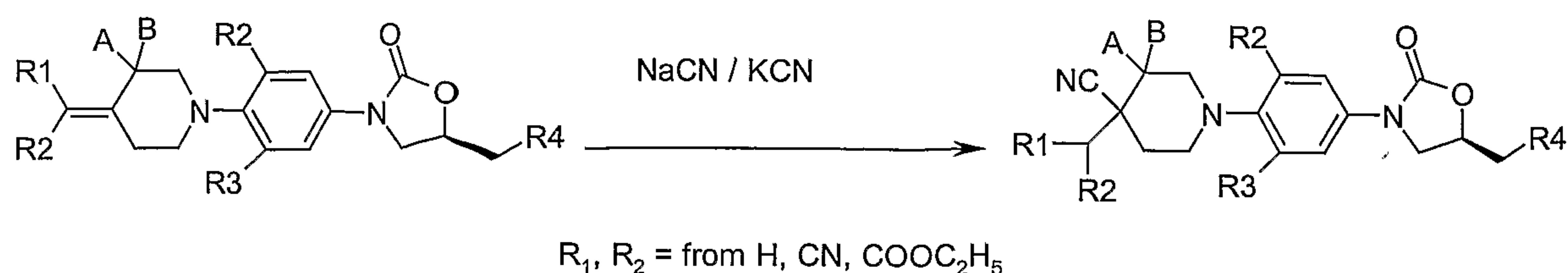
Scheme-16
