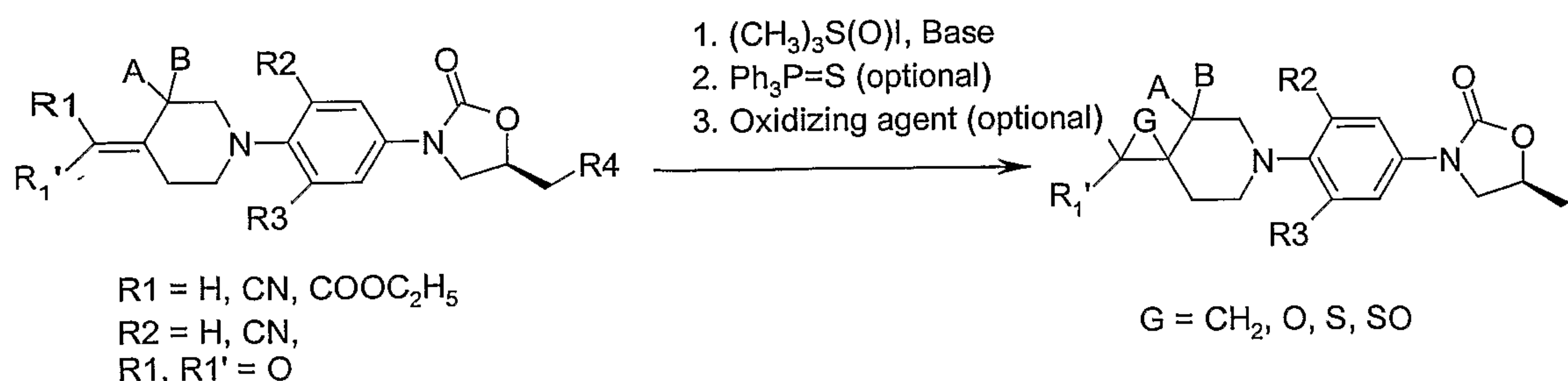
Scheme-1
