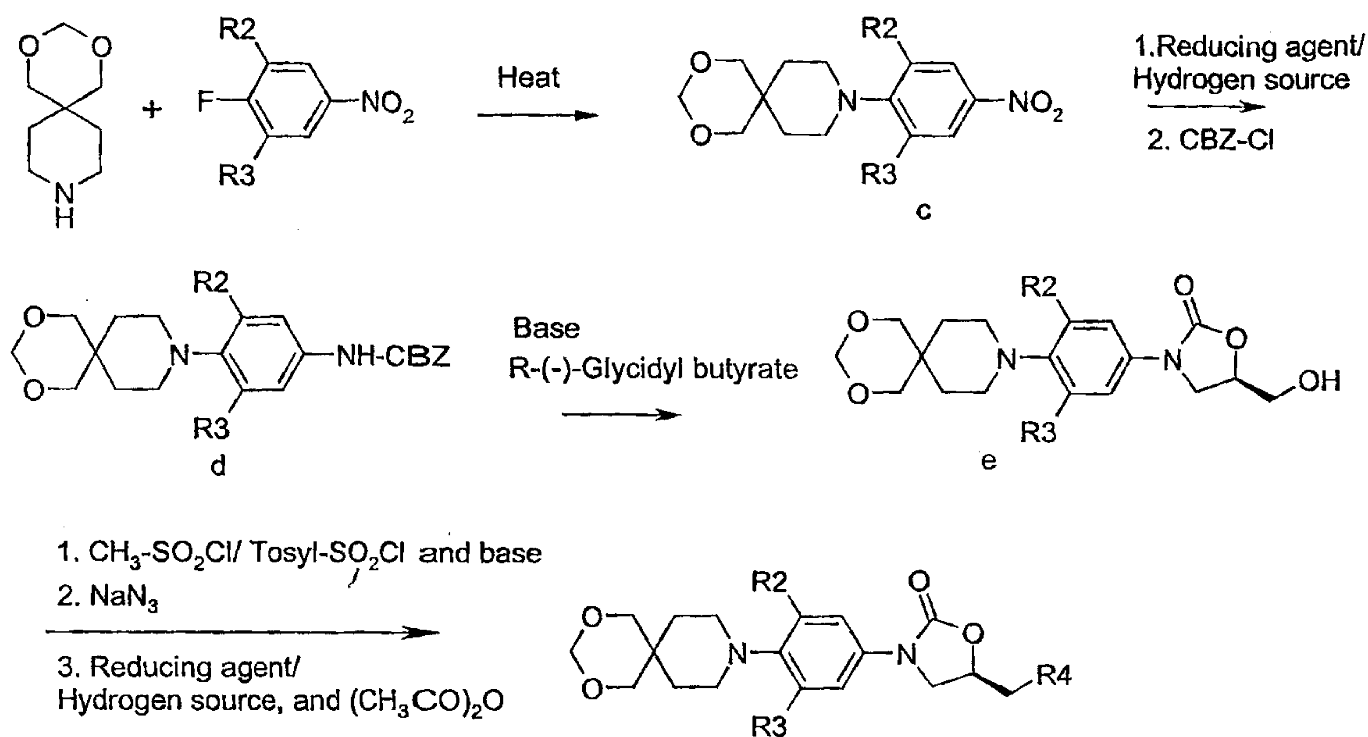
Scheme-6
