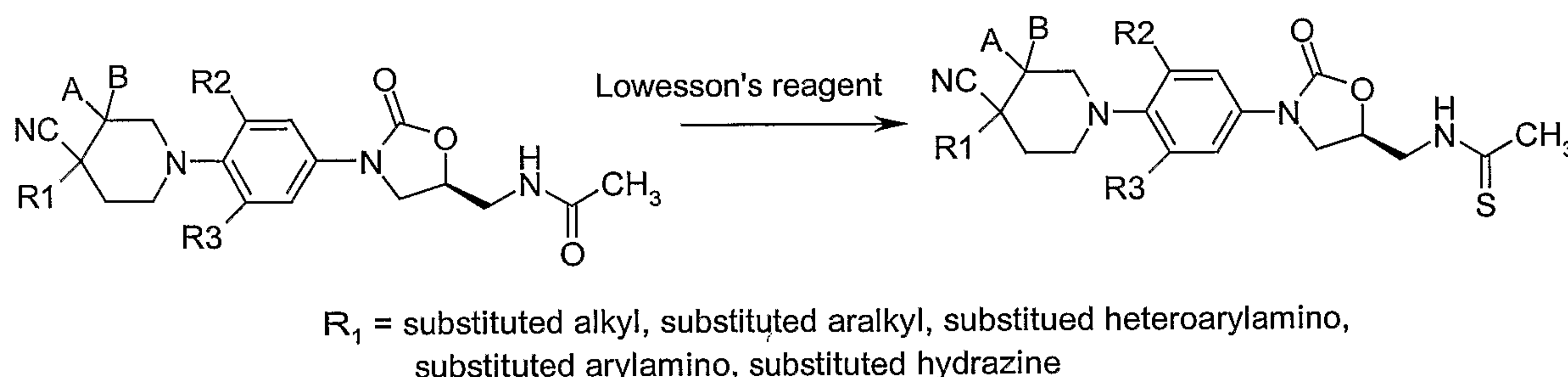
Scheme-19
