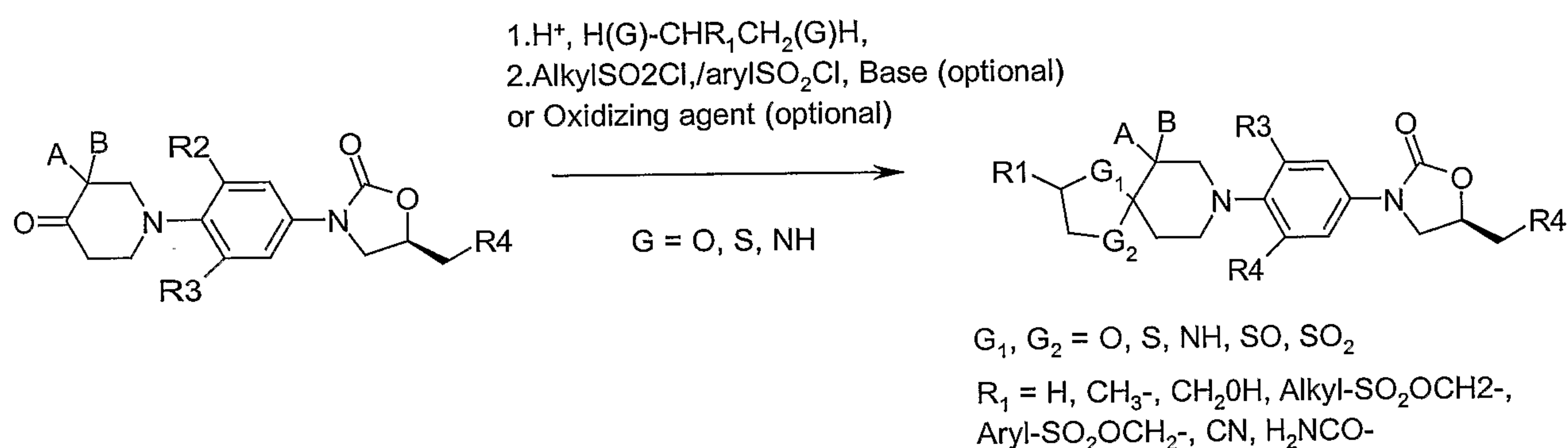
Scheme-3
