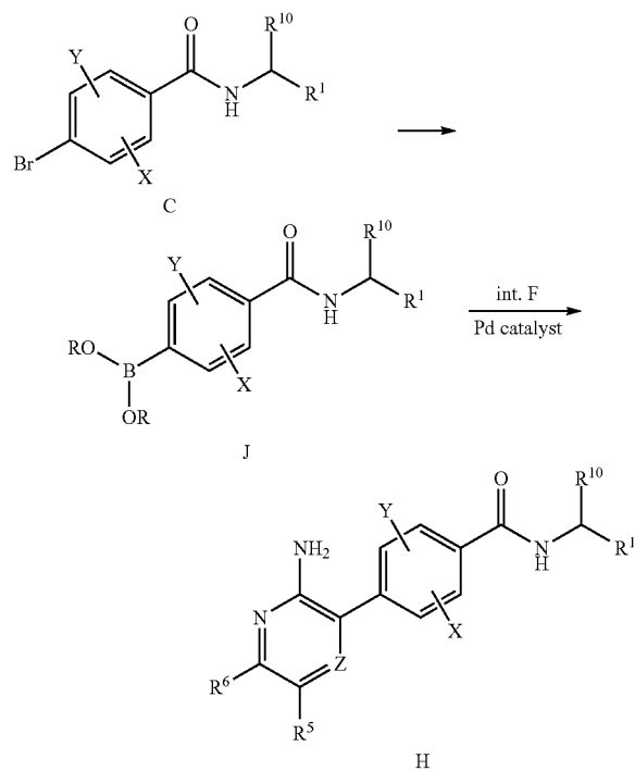
Scheme B.
