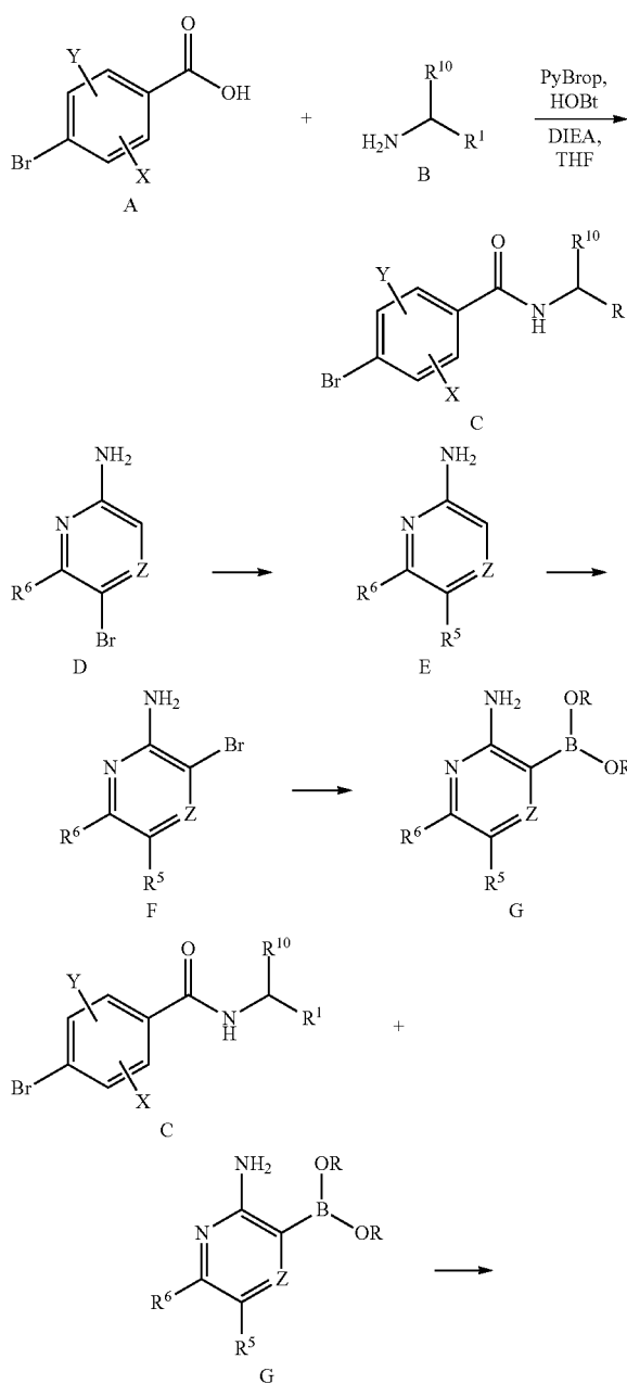
Scheme A.
