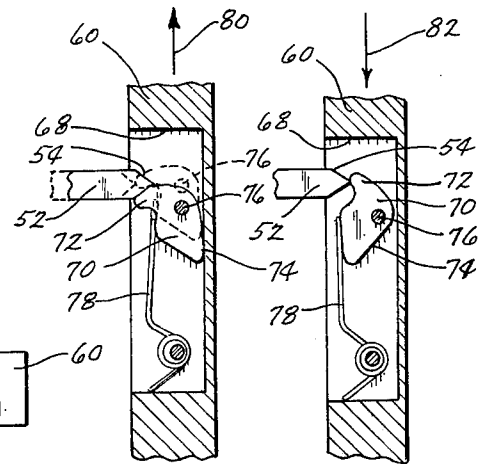
Fig. 6 Fig. 7
