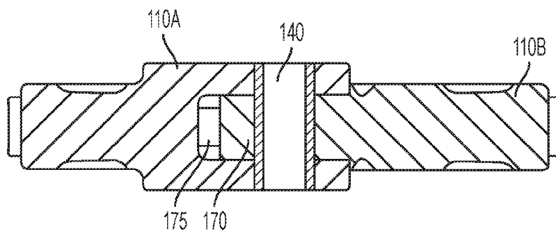
SECTION A-A FIG. 3B
