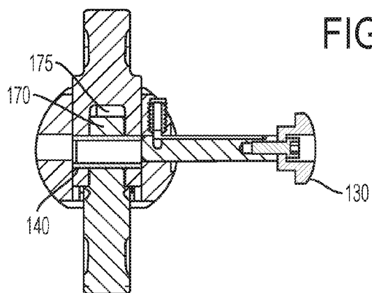
SECTION H-H FIG. 9C
