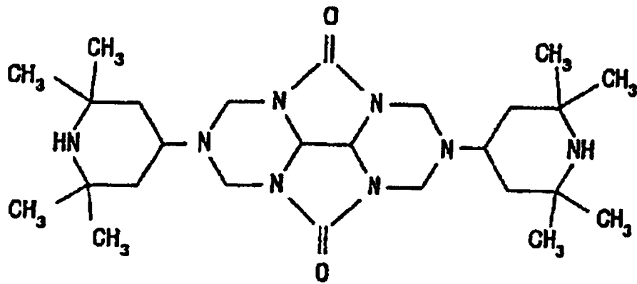
Composé 4
