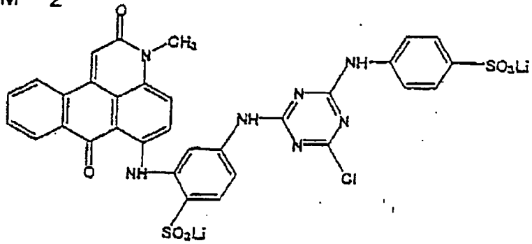
M-2
