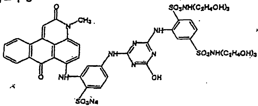
M-10
