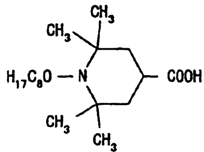
Verbindung 12
