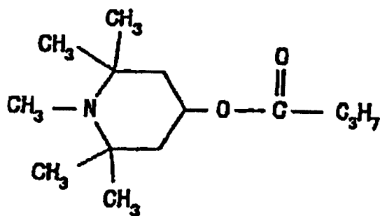
Composé 3
