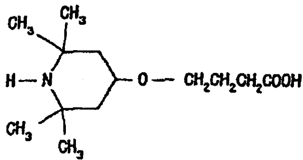
Composé 15
