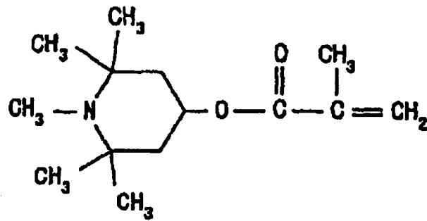
Composé 5
