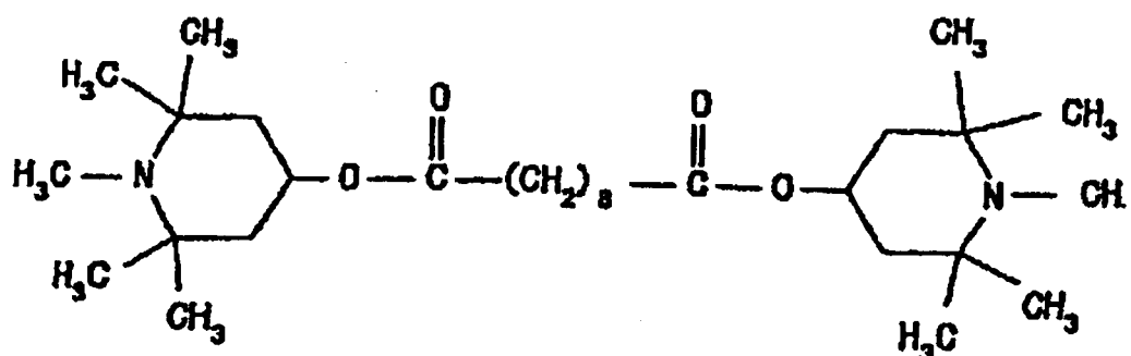
Composé 7
