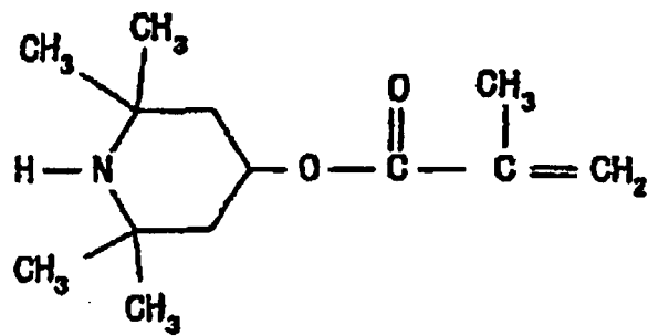
Composé 6
