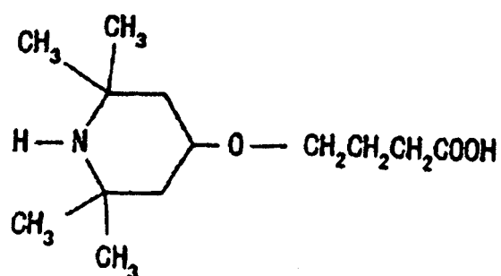
Verbindung 15
