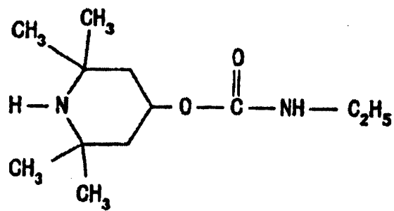
Verbindung 10
