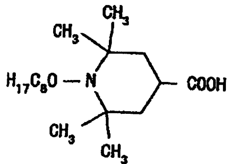
Composé 12
