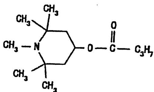
Verbindung 3
