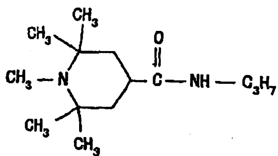
Composé 9
