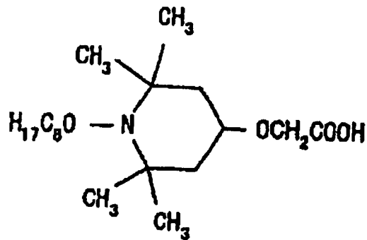
Composé 1
