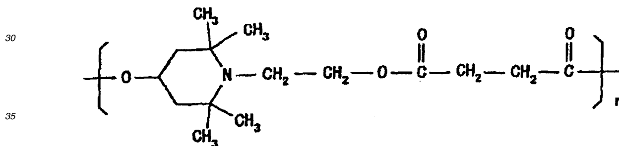
Composé 17
