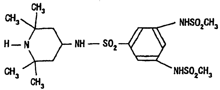
Verbindung 8
