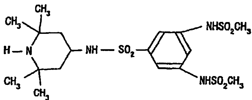
Composé 8
