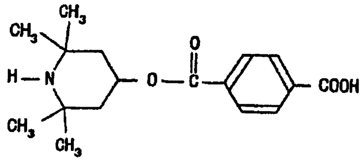
Composé 13
