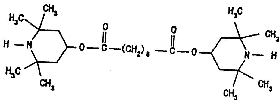
Verbindung 2
