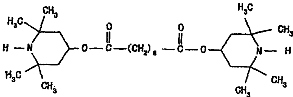
Composé 2
