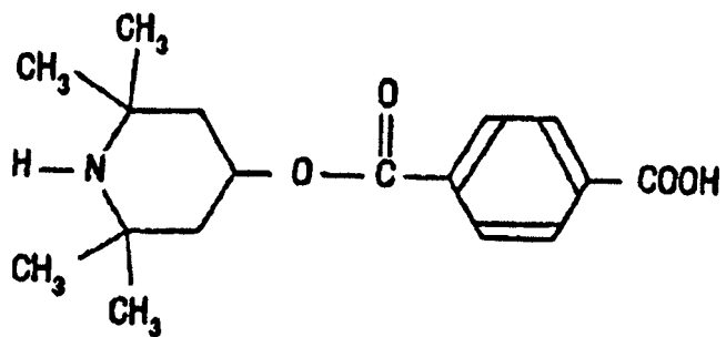
Verbindung 13
