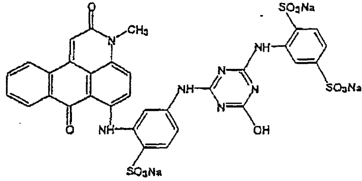
M-1
