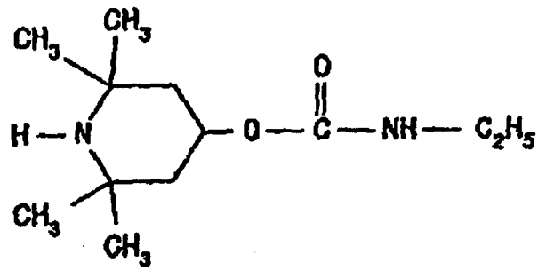
Composé 10
