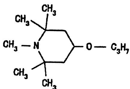
Verbindung 14
