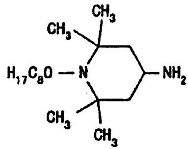
Verbindung 11
