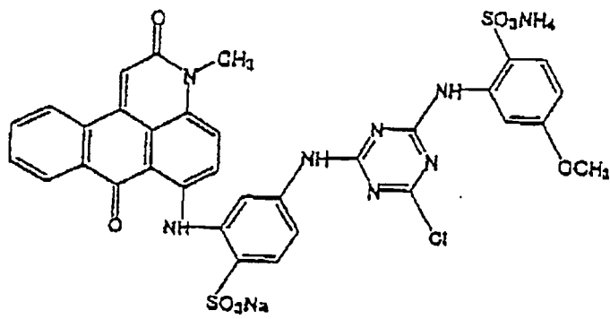
M-9
