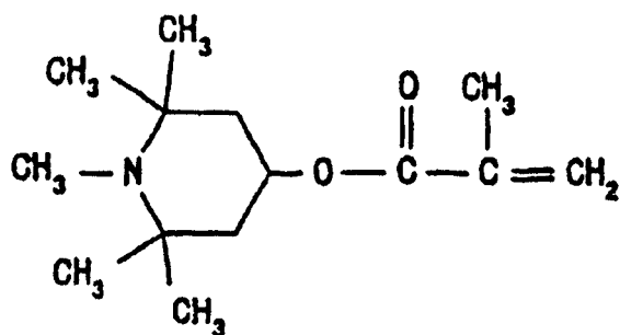
Verbindung 5
