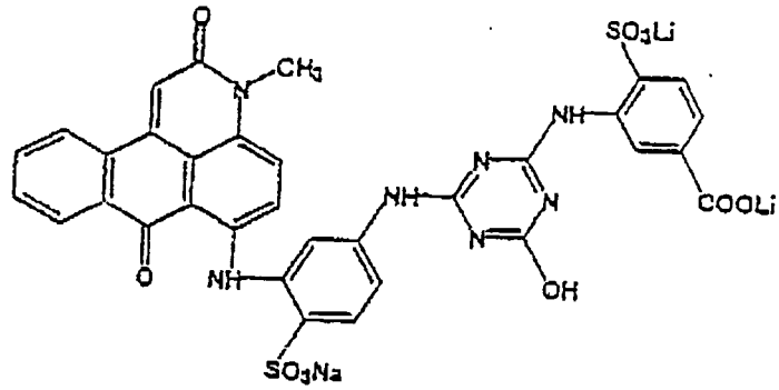
M-7
