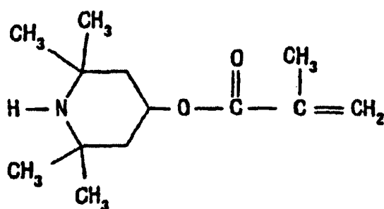
Verbindung 6
