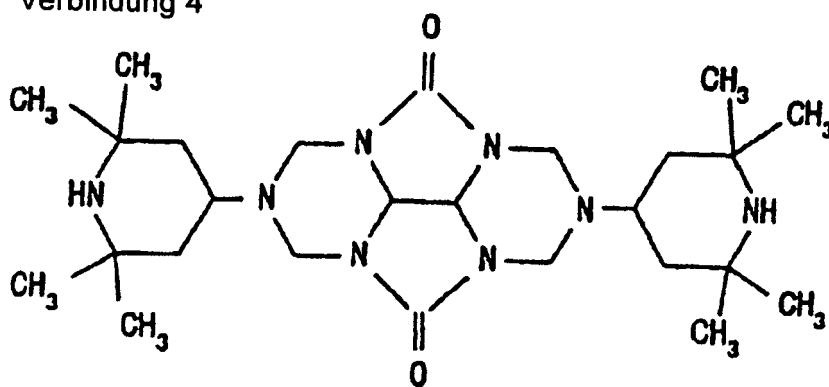
Verbindung 4
