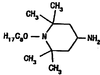
Composé 11
