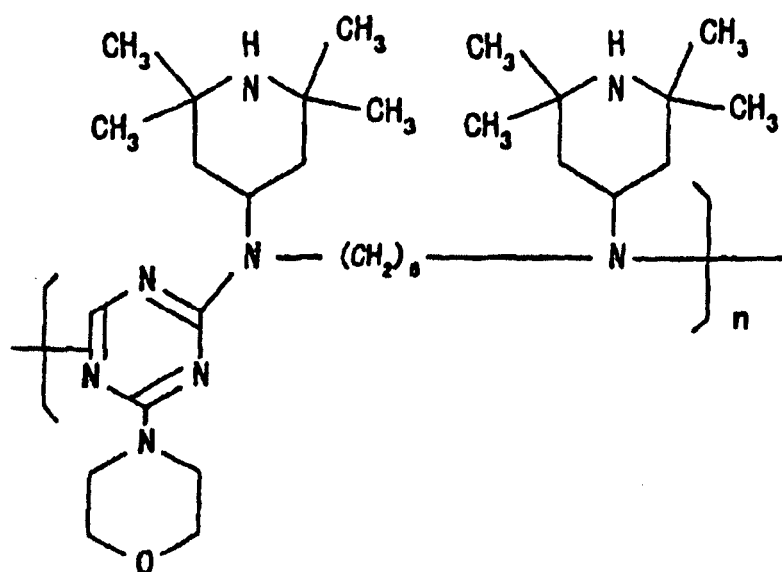
Verbindung 16
