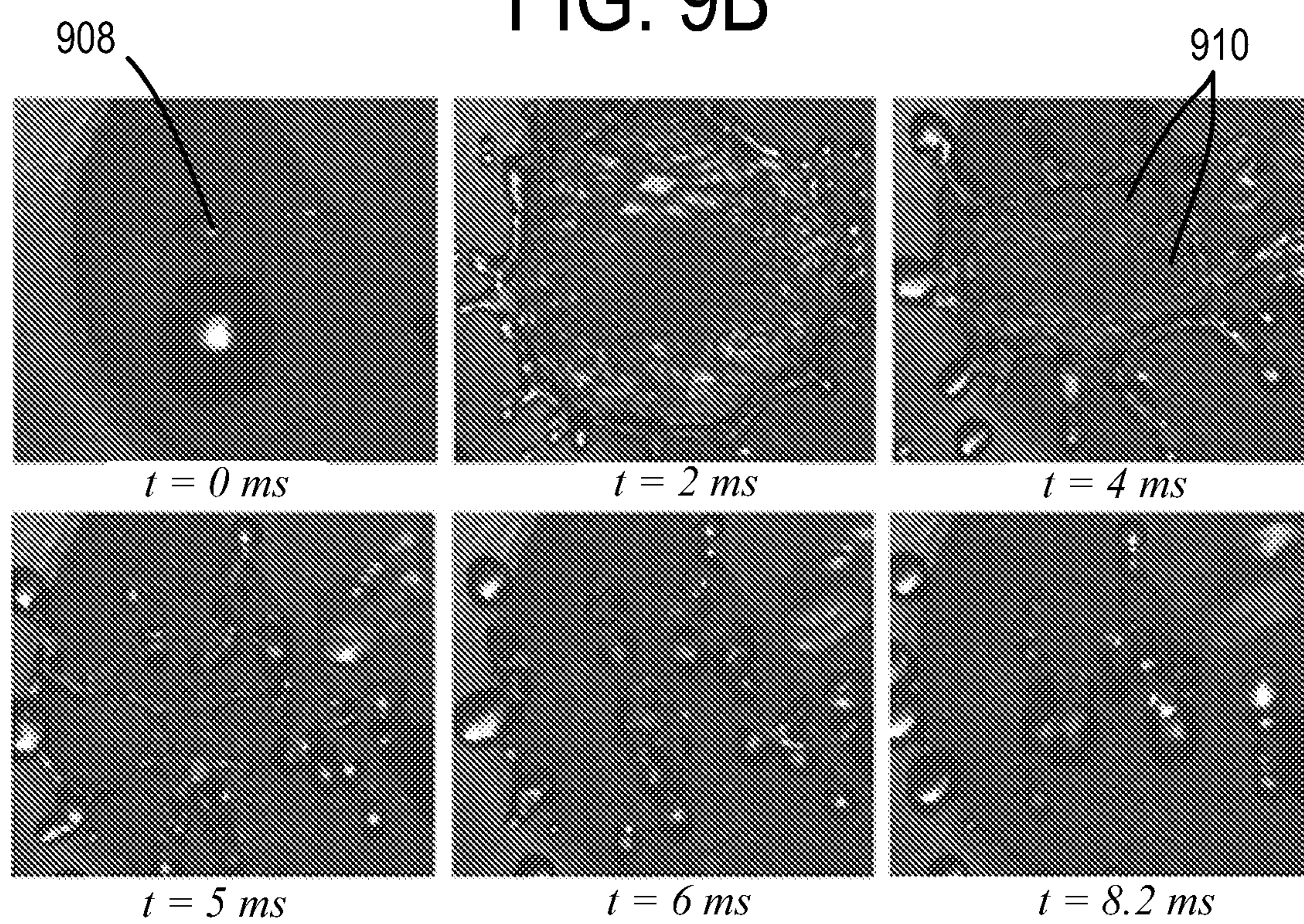
FIG. 9C
