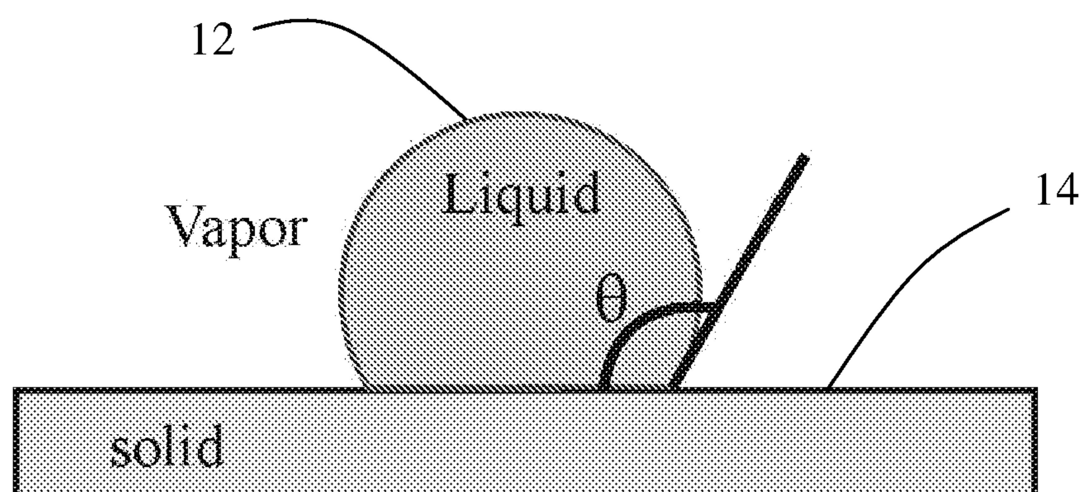
FIG. 1a
