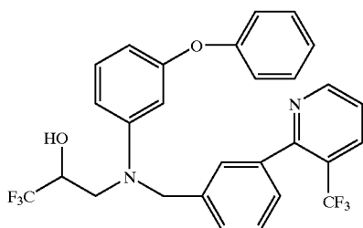
3-[(3-phenoxyphenyl)[[3-(3-trifluoromethyl)-2-pyridinyl]phenyl]methyl]amino]-1,1,1-trifluoro-2-propanol
