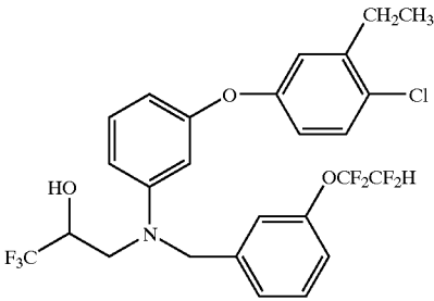
3-[[3-(4-chloro-3-ethylphenoxy)phenyl]-[[3-(1,1,2,2-tetrafluoroethoxy)phenyl]methyl]amino]-1,1,1-trifluoro-2-propanol
