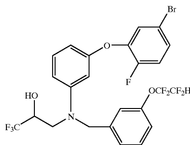
3-[[3-(5-bromo-2-fluorophenoxy)phenyl][[3-(1,1,2,2-tetrafluoroethoxy)phenyl]methyl]amino]-1,1,1-trifluoro-2-propanol
