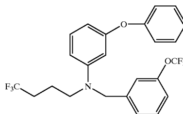
N-(3-phenoxyphenyl)-N-(4,4,4-trifluorobutyl)-3-(trifluoromethoxy)benzenemethanamine
