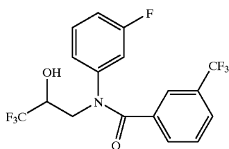
N-(3-fluorophenyl)-N-(3,3,3-trifluoro-2-hydroxypropyl)-3-(trifluoromethyl)benzamide
