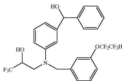
\alpha -Phenyl-3-[[[3-(1,1,2,2-tetrafluoroethoxy)phenyl]methyl](3,3,3-trifluoro-2-hydroxypropyl)benzenemethanol
