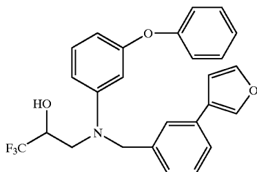
3-[(3-phenoxyphenyl)[[3-(3-furanyl)phenyl]methyl]amino]-1,1,1-trifluoro-2-propanol
