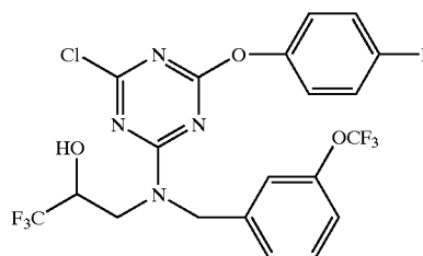
N-[2-chloro-6-(p-fluorophenoxy)-1,3,5-triazin-4-yl]-3-[[[3-(trifluoromethoxy)phenyl]methyl]amino]-1,1,1-trifluoro-2-propanol
