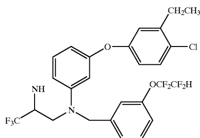
3-[[3-(4-chloro-3-ethylphenoxy)phenyl]-[[3-(1,1,2,2-tetrafluoroethoxy)phenyl]methyl]amino]-1,1,1-trifluoro-2-propanamine
