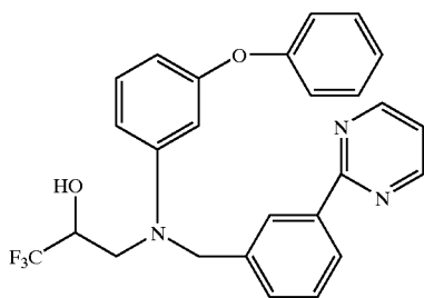
3-[(3-phenoxyphenyl)[[3-(2-pyrimidinyl)phenyl]methyl]amino]-1,1,1-trifluoro-2-propanol
