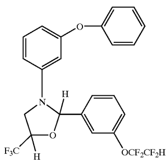
3-(3-phenoxyphenyl)-2-[3-(1,1,2,2-tetrafluoroethoxy)phenyl]-5-(trifluoromethyl) oxazolidine
