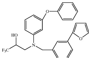
3-[(3-phenoxyphenyl)[[3-(2-furanyl)phenyl]methyl]amino]-1,1,1-trifluoro-2-propanol
