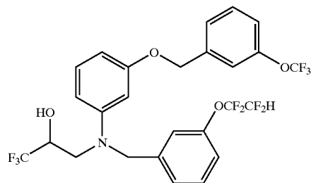
3-[[[3-(1,1,2,2-tetrafluoroethoxy)phenyl]methyl][3-(trifluoromethoxy)phenyl]-methoxy]phenyl]amino]-1,1,1-trifluoro-2-propanol
