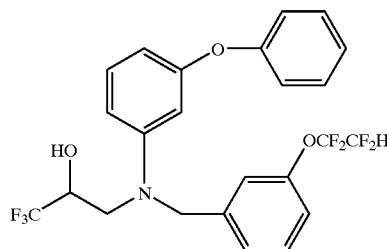
3-[[3-(3-phenoxyphenyl)(3-(1,1,2,2-tetrafluoroethoxy)phenyl)methyl]amino]-1,1,1-trifluoro-2-propanol
