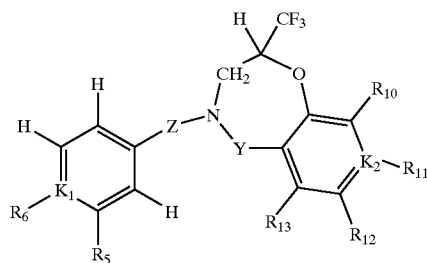
Cyclo-VII
