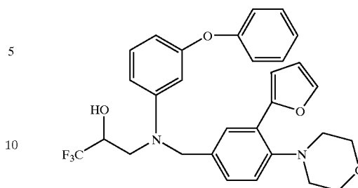
3-[(3-phenoxyphenyl)[[3-(2-furanyl)-4-(4-morpholinyl)phenyl]methyl]amino]-1,1,1-trifluoro-2-propanol
