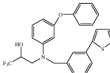
3-[(3-phenoxyphenyl)[[3-(2-thienyl)phenyl]methyl]amino]-1,1,1-trifluoro-2-propanol
