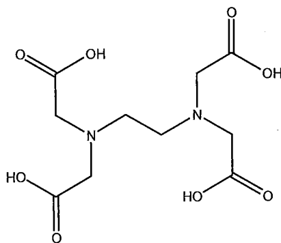
Ethylene glycol bis(2-aminoethyl) tetracetic acid CAS 60-00-4
