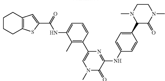
GDC-0834
