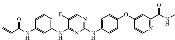
CNX-774
