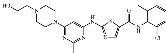
Dasatinib
