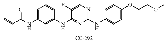
CC-292
