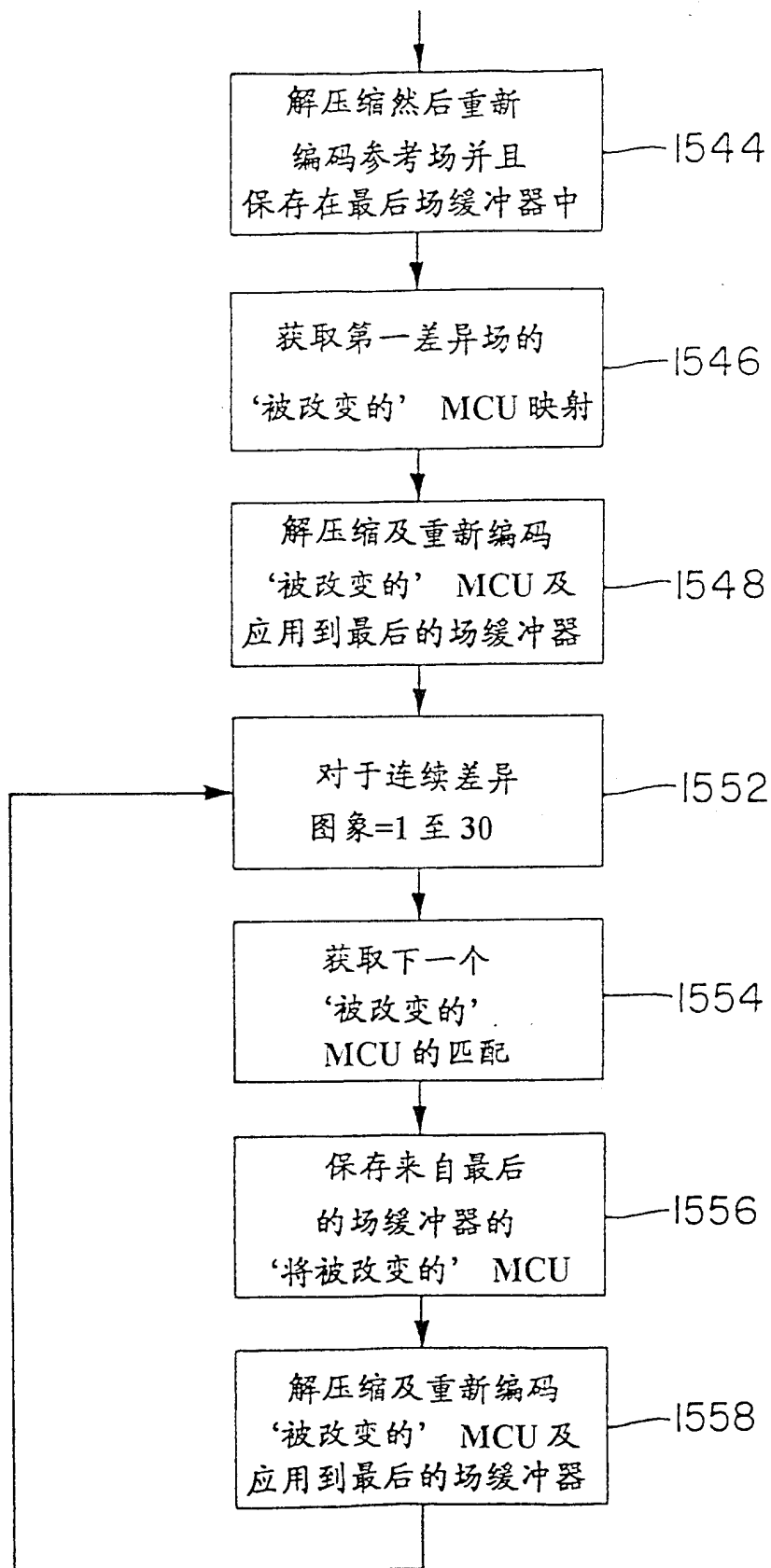
图 66 建立后向历史缓冲器
