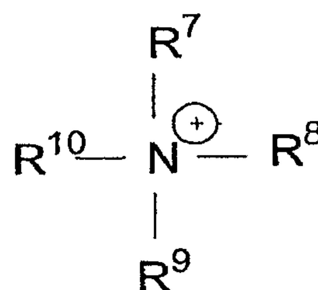
Ammonium
