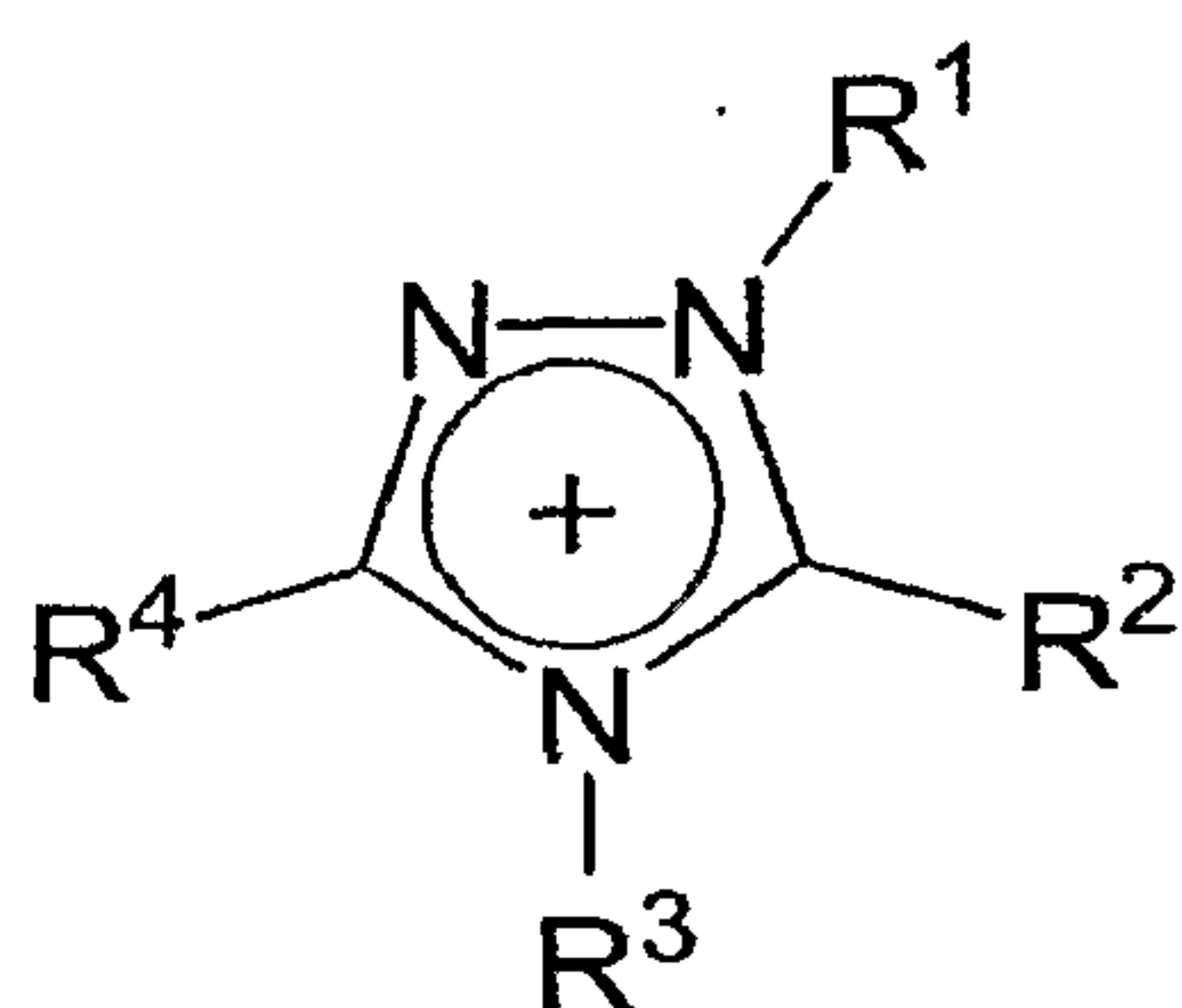
Triazolium
