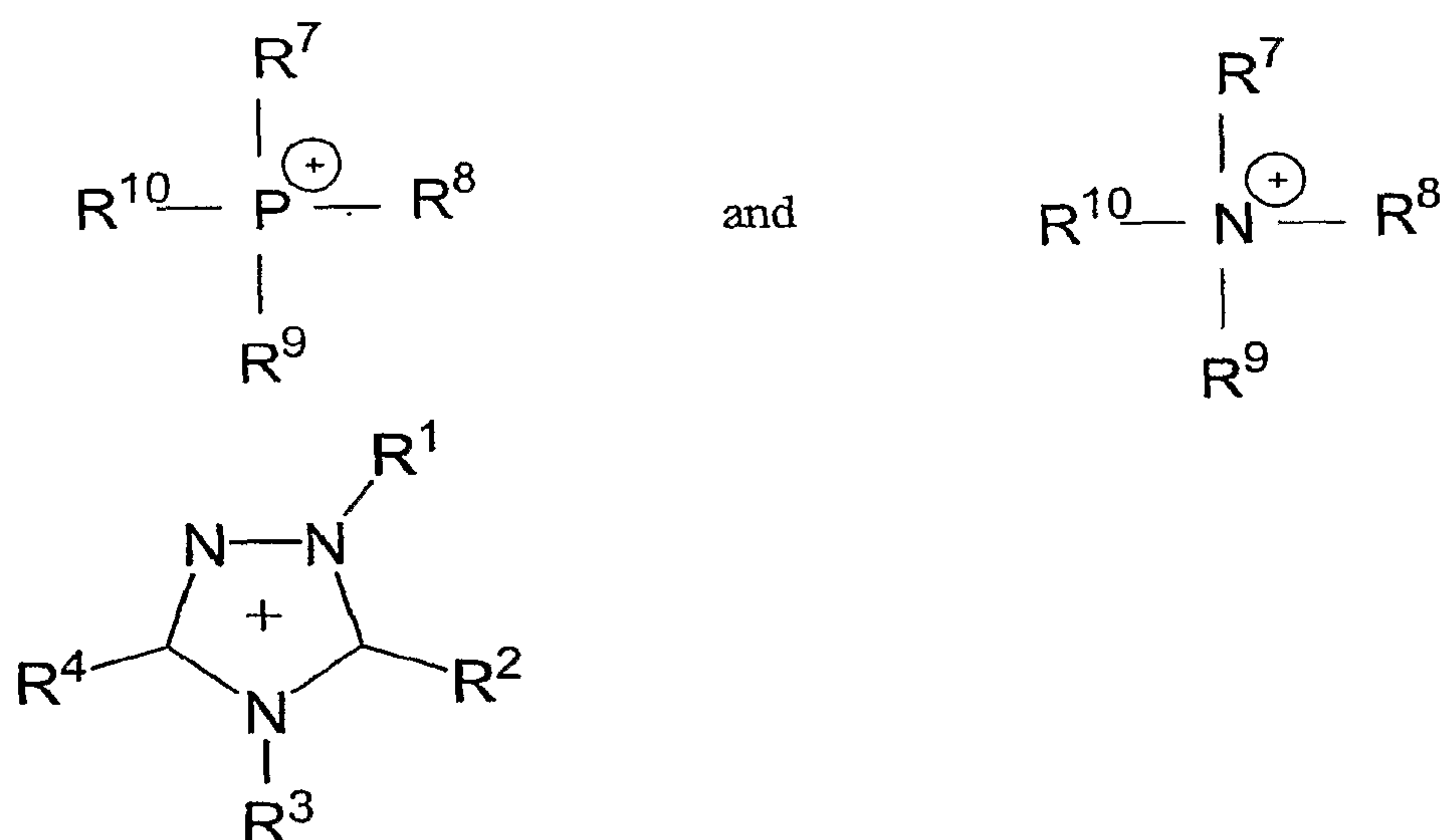
Triazolium
