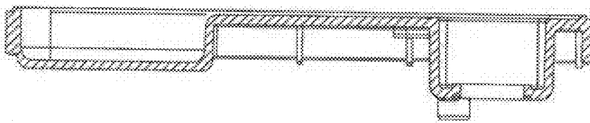
SECTION D-D
