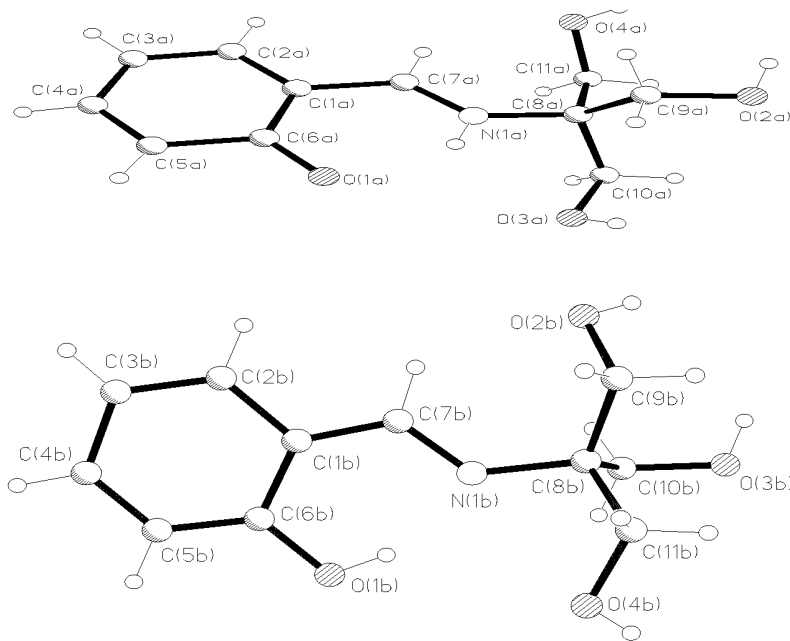
Fig. 1. Structura moleculei I
