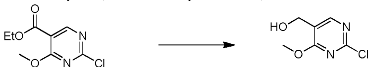
Etapa 2: (2-clor-4-metoxipirimidin-5-il)metanol
