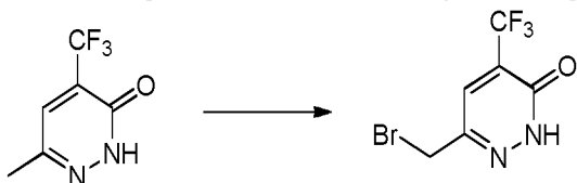
Etapă 1: 6-(brommetil)-4-(trifluormetil)piridazin-3(2H)-onă
