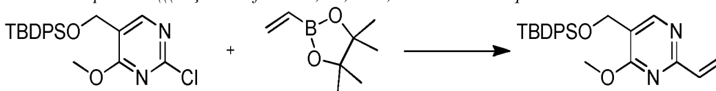
Etapa 4: 5-(((terț-butildifenilsilil)oxi)metil)-4-metoxi-2-vinilpirimidină
