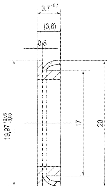
Section A-A 3:1
