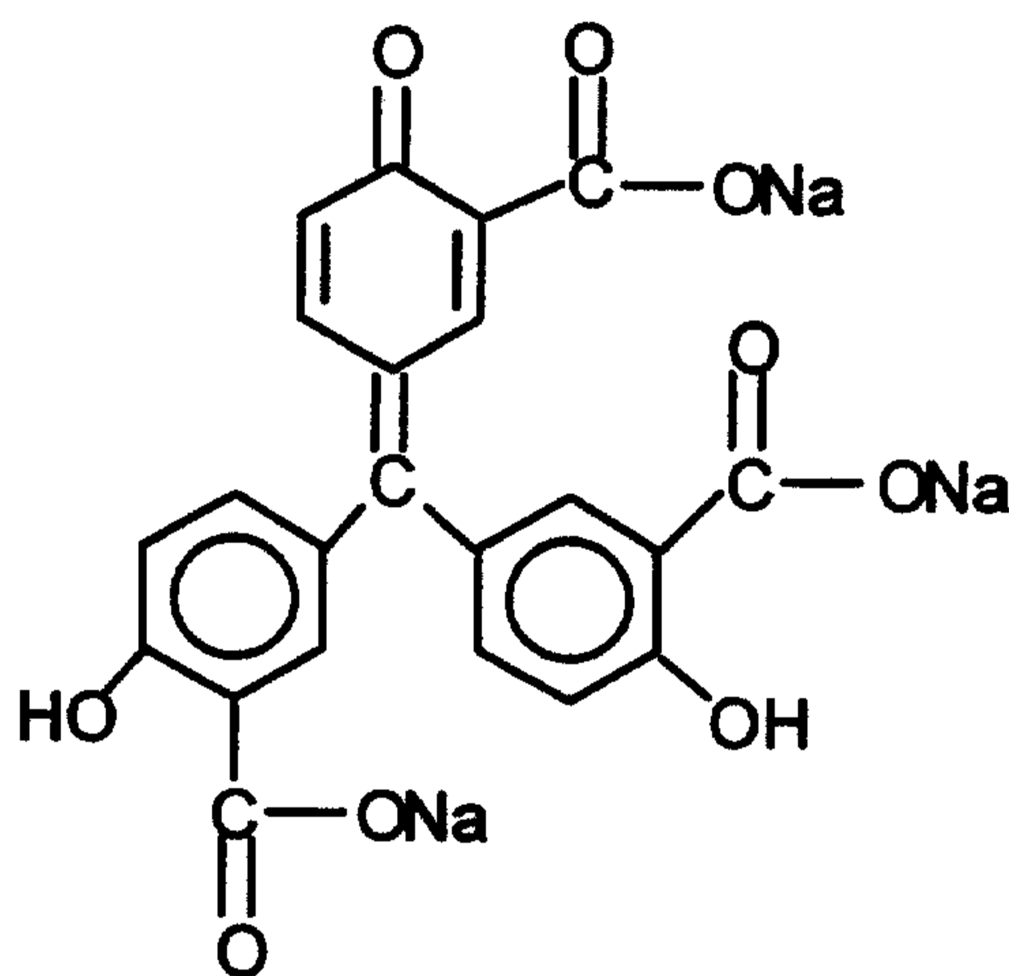
Trisodium Salt
