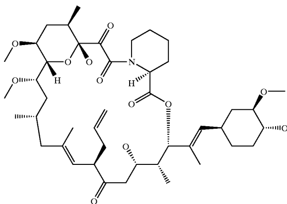
Tacrolimus
