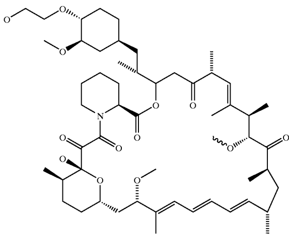
Everolimus
