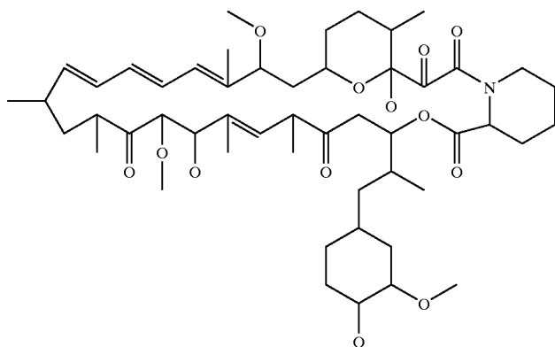
Sirolimus
