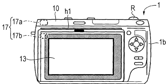
도면3b
