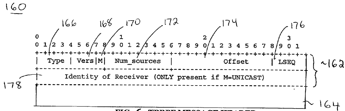
FIG. 6 TBRPF MESSAGE HEADER
