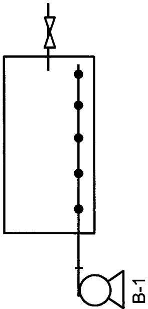
FIG. 16A
