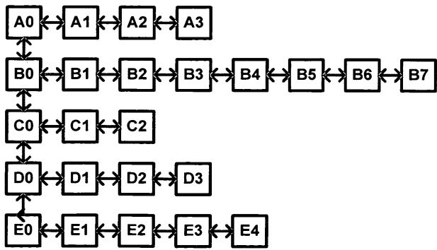
데이터 구조
