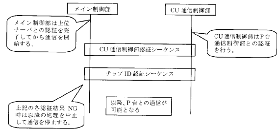
(b) 遊技機電源起動時認証シーケンス
