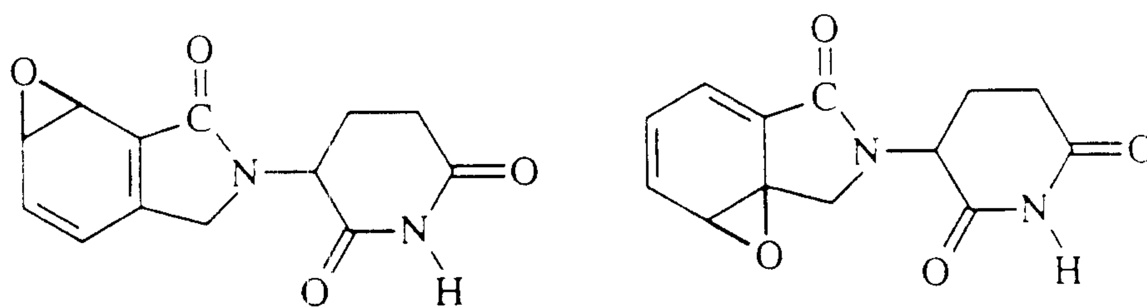
Epoxides of EM 12
