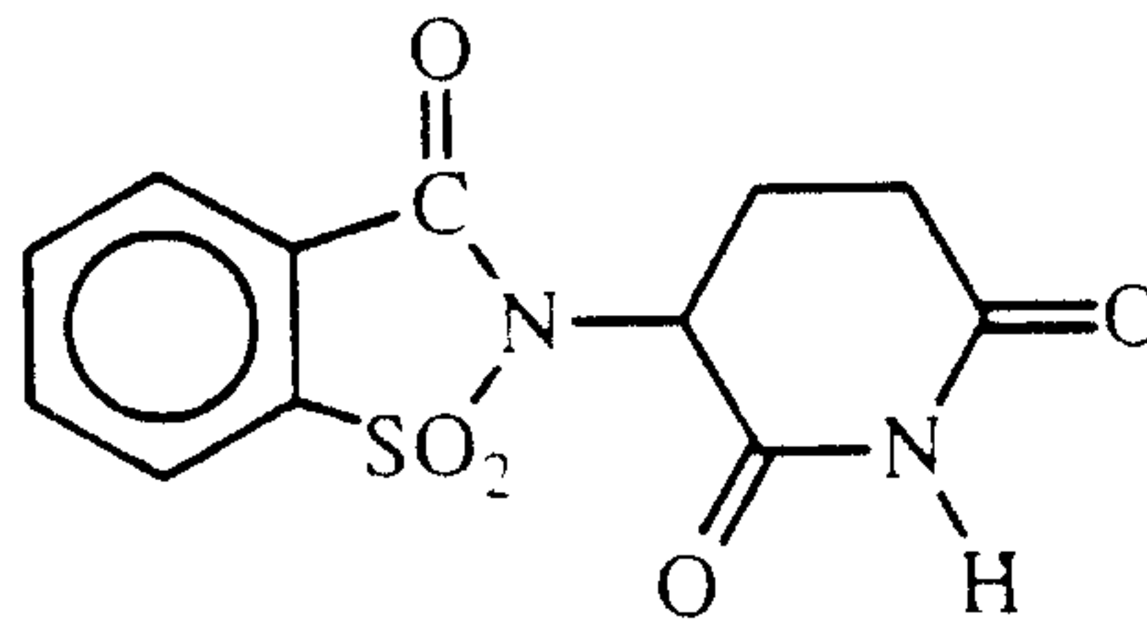
supidimide.
