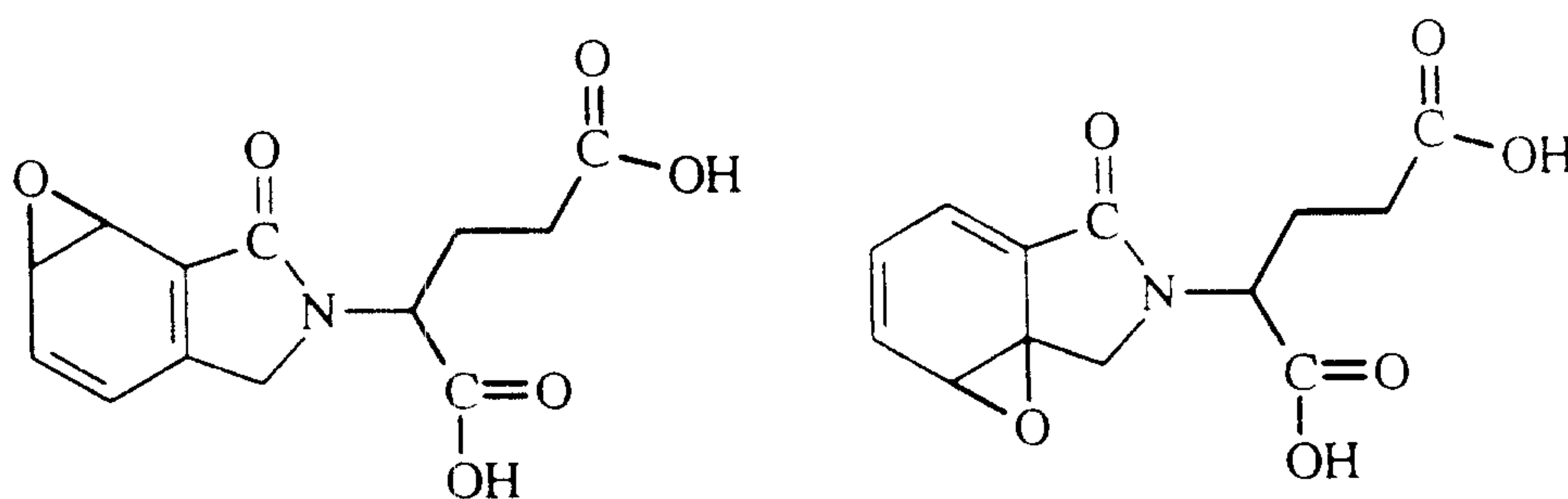
Epoxides of EM 138
