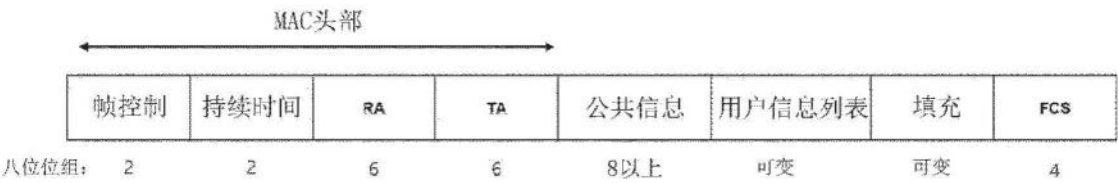
触发帧格式
