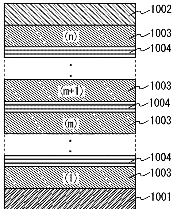
FIG. 21B
