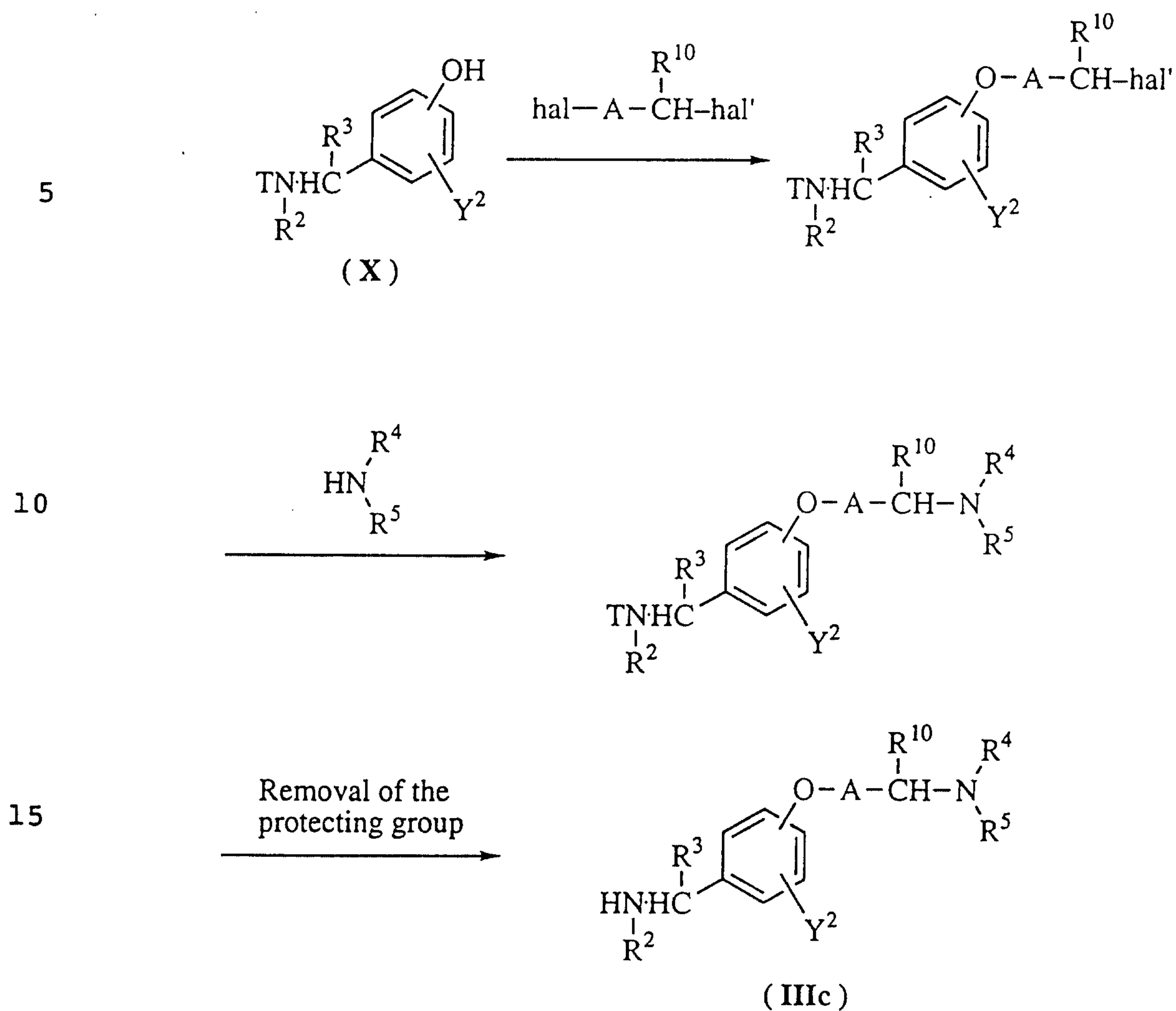
Scheme (D)
