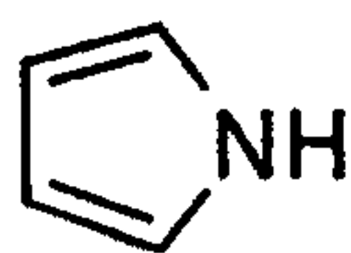
pyrrole (pyrrolyl)
