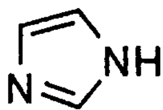
imidazole (imidazolyl)
