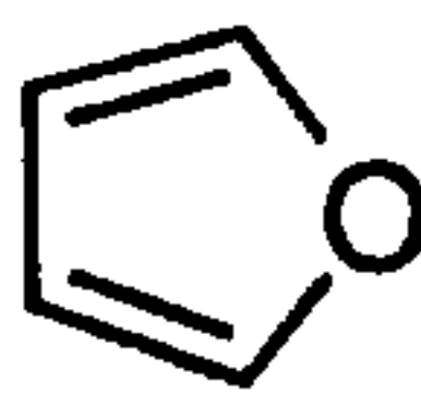
furan (furyl)
