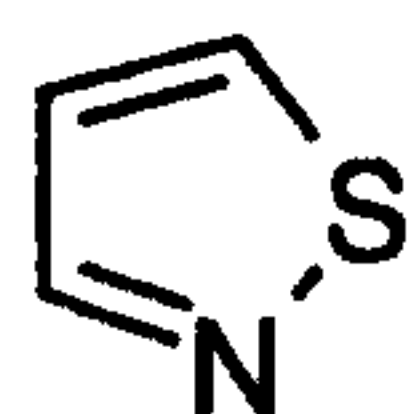
isothiazole (isothiazolyl)
