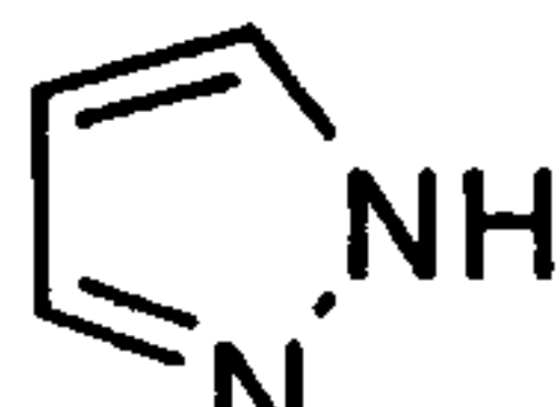
pyrazole (pyrazolyl)
