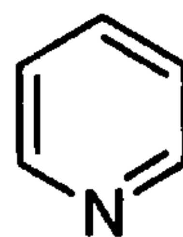
pyridine (pyridinyl)
