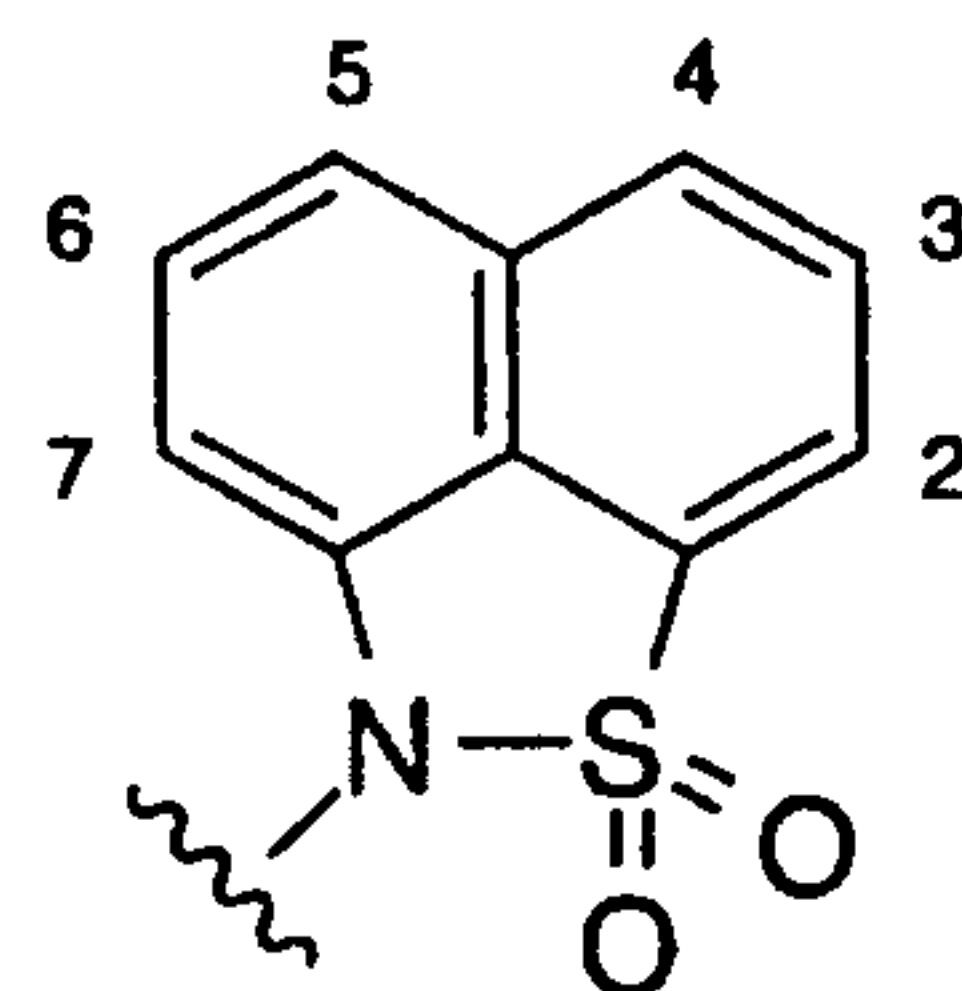
1,8-naphthosultamyl
