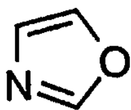
oxazole (oxazolyl)
