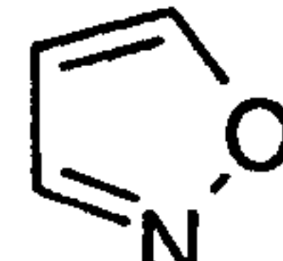
isoxazole (isoxazolyl)
