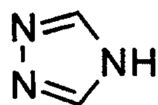
triazole (triazolyl)
