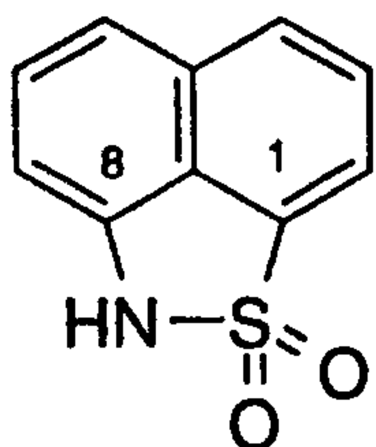
1,8-naphthosultam
