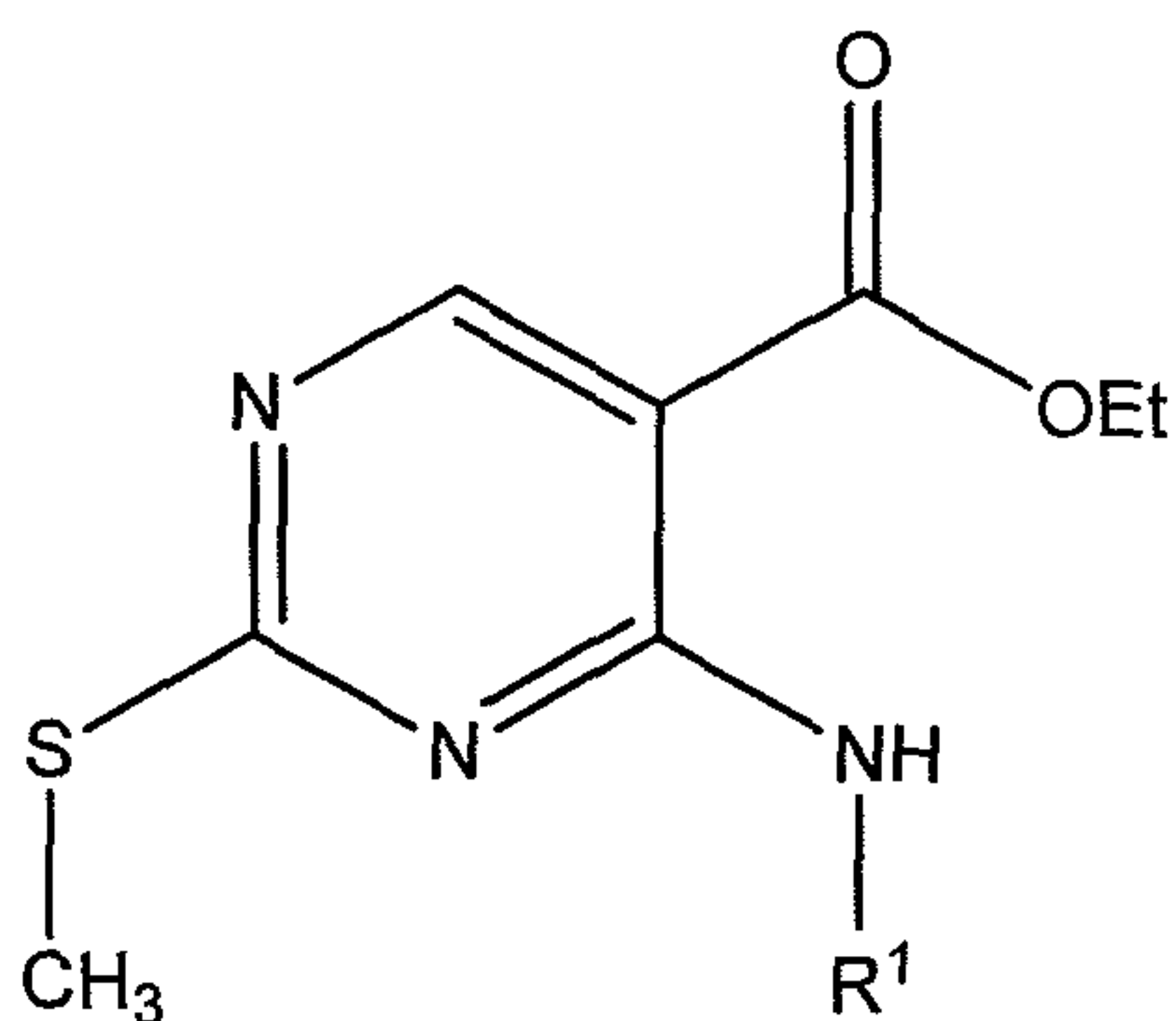
Formula VI.
