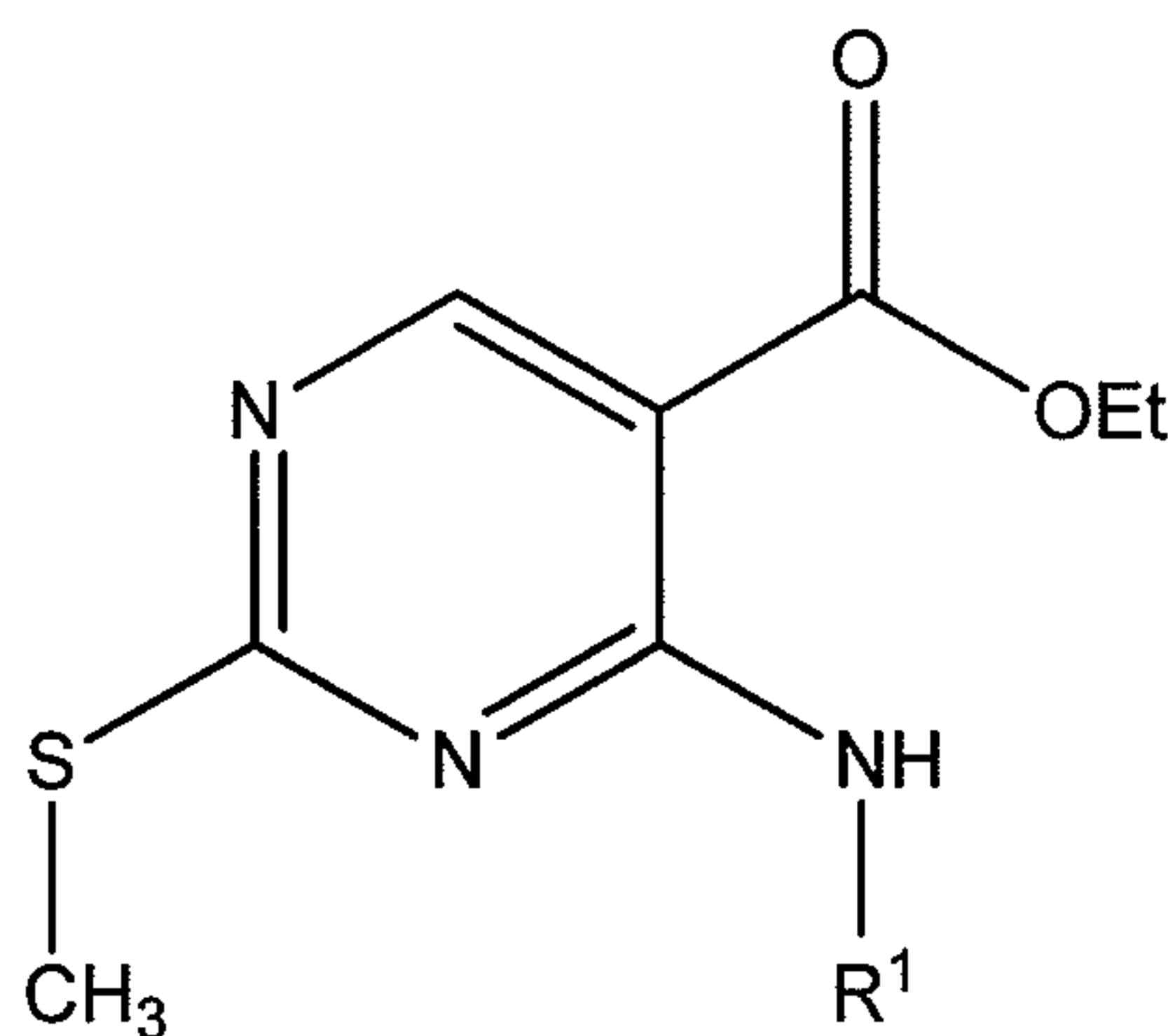
Formula VI.
