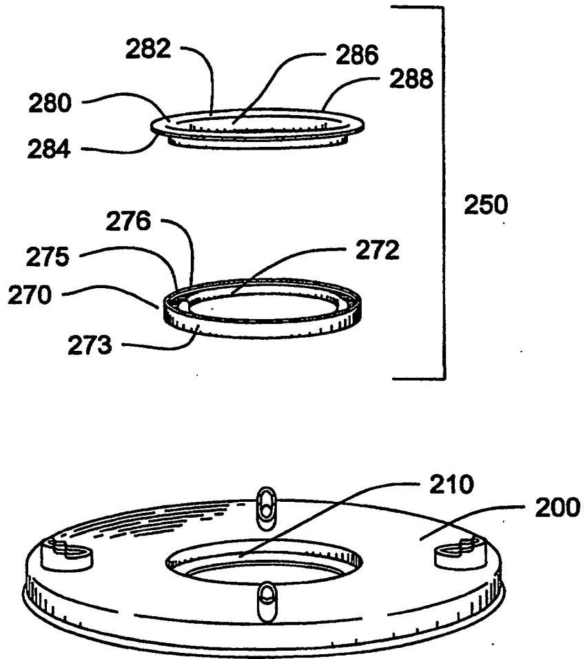
FIG. 8c
