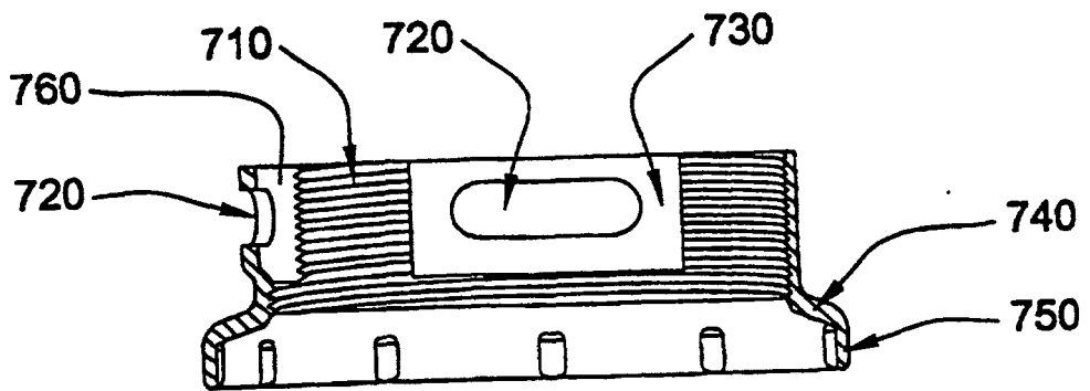
FIG. 14b
