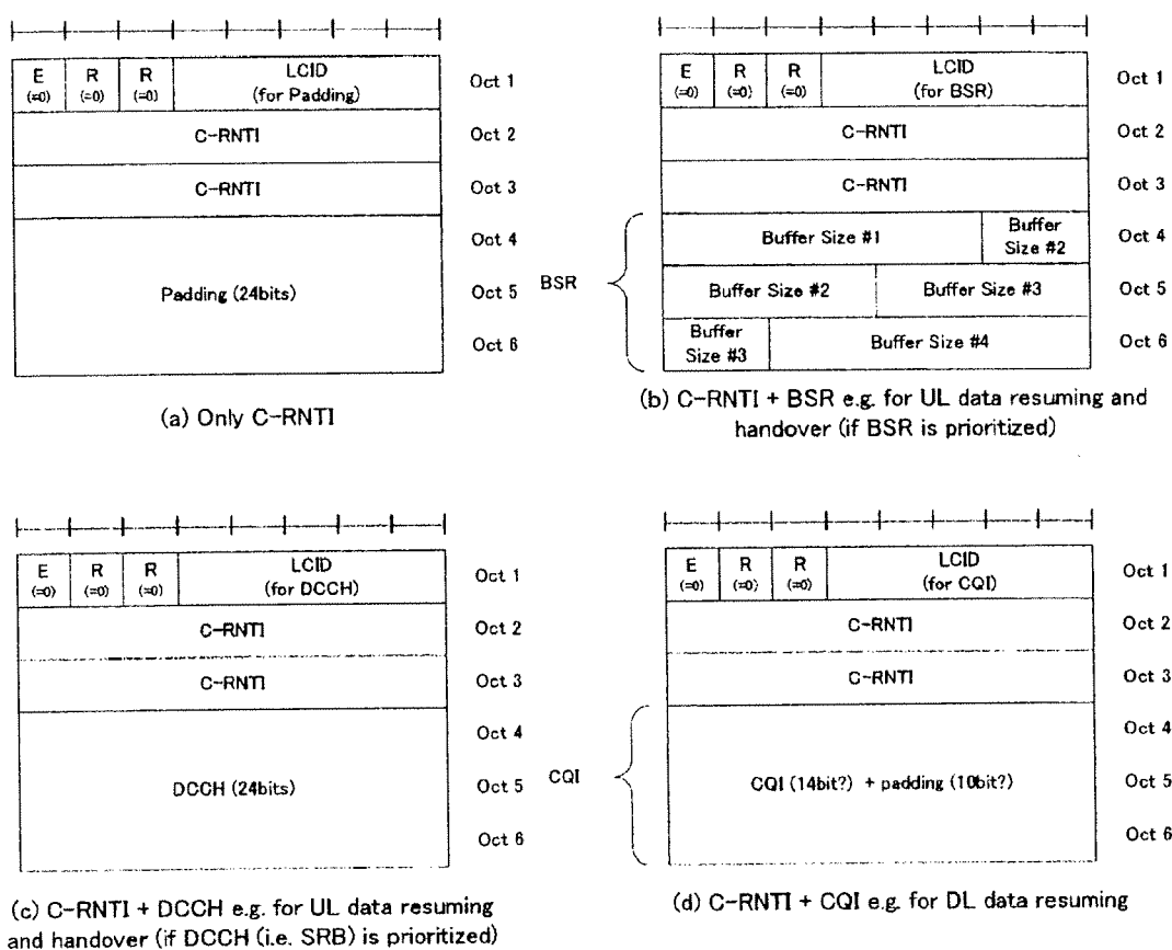
FIG. 31
