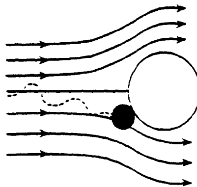
d) Diffusion
