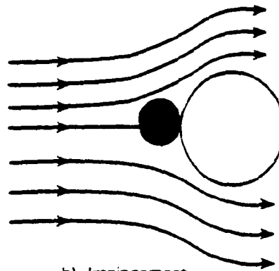
b) Impingement
